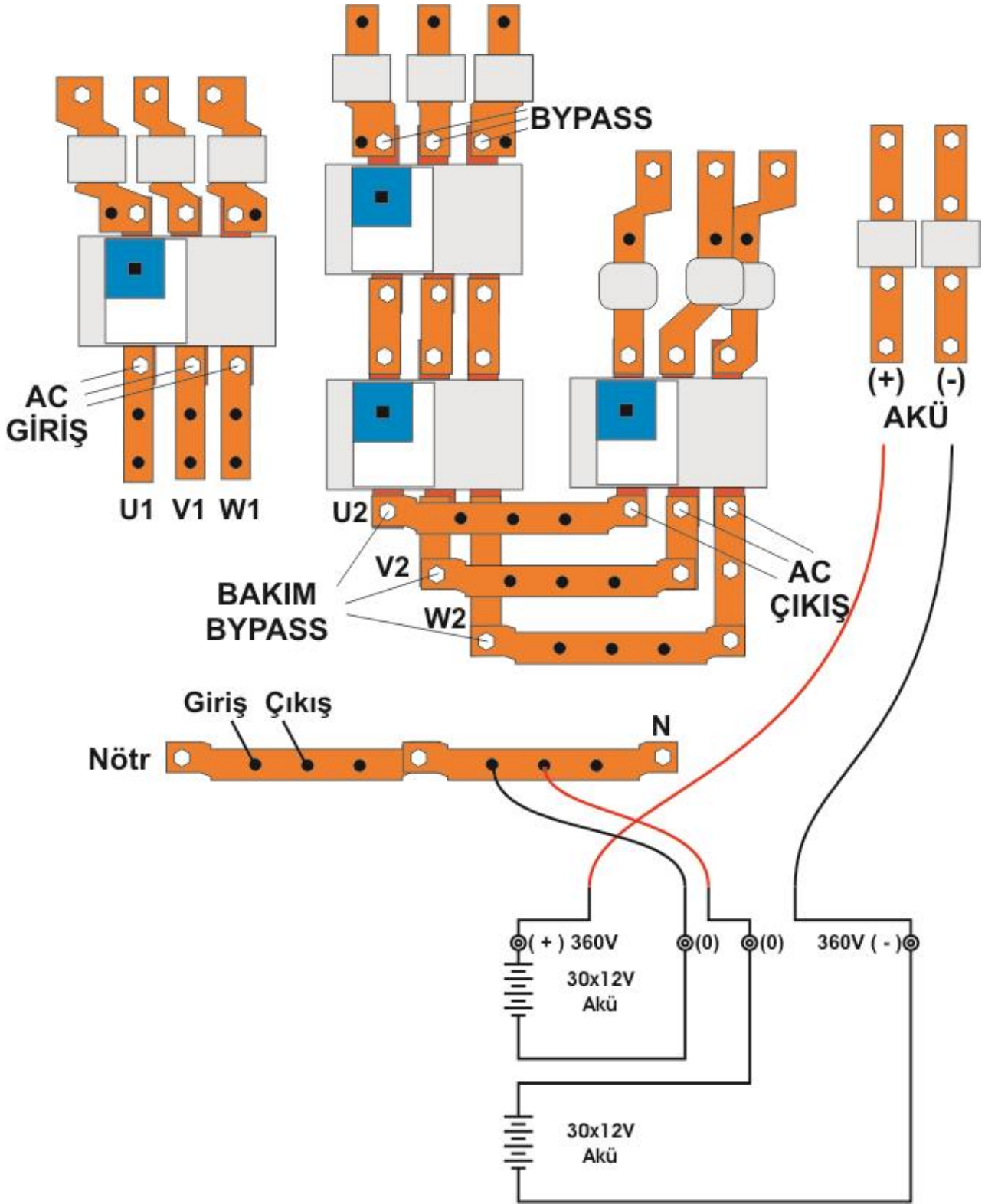
Şekil 2.2 200-250-300-350-400-450-500kVA Kablo Bağlantısı
