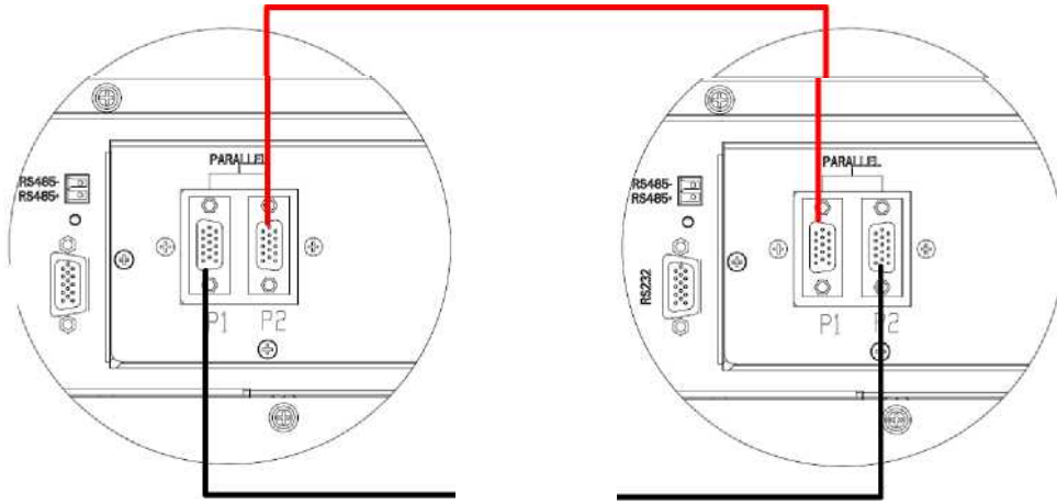
Şek.3- 3: "1+N" Sistemi Paralel Kabloların Bağlantısı
