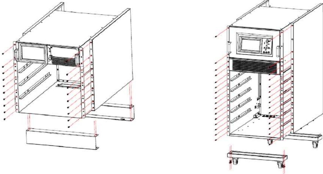
(a) Yan panelleri ve tespit parçalarını sökün
