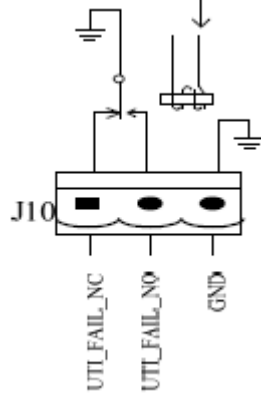
Şek.1- 13: Elektrik Kesinti Uyarısı Kuru Kontaktörü
