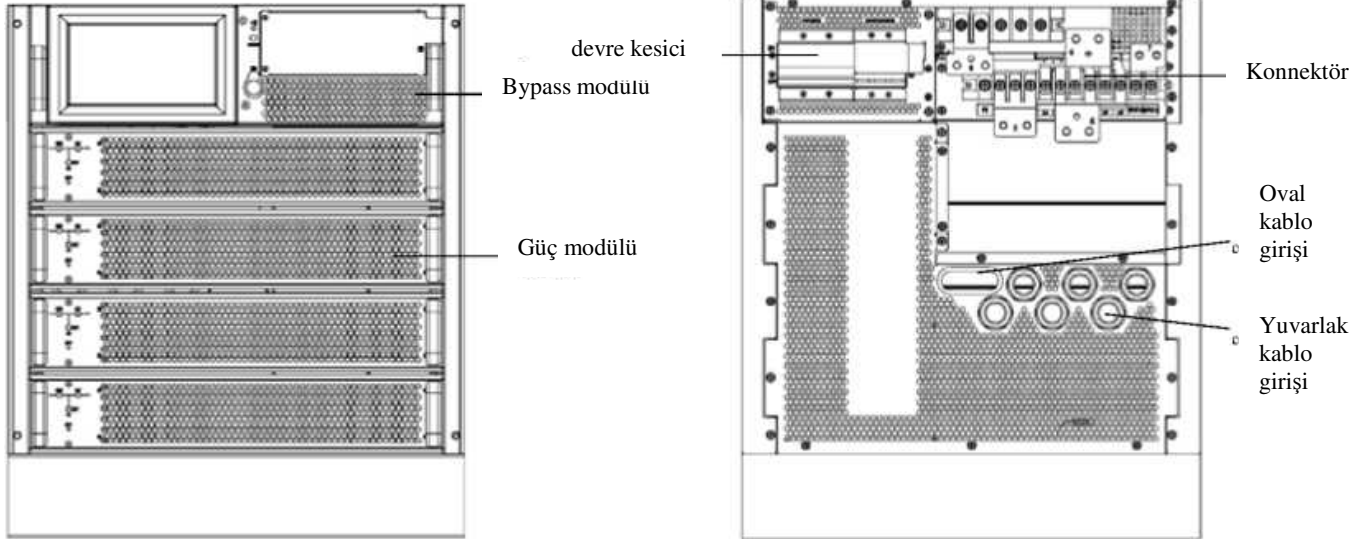
(b) 4 modüllü kabin
