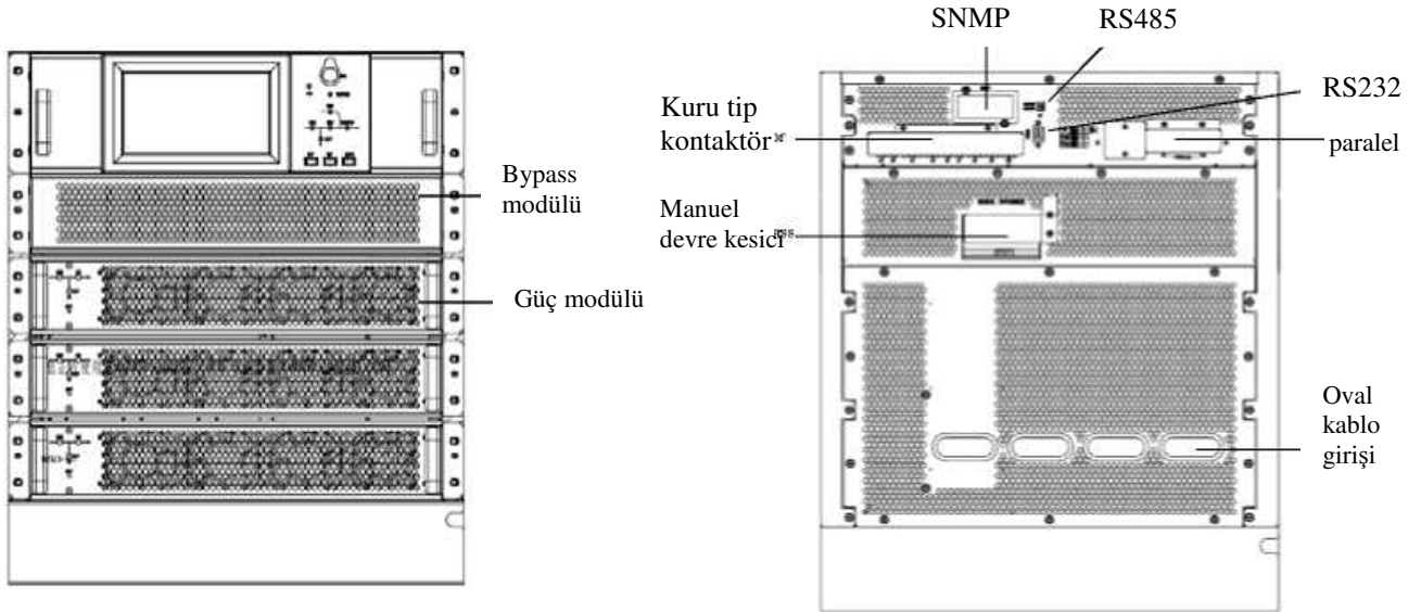
(c) 3 modüllü kabin
