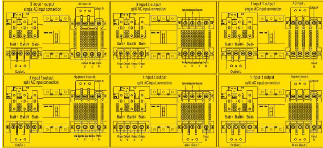
Şekil B-2: 6 Yuvalı kabinin Güç Bağlantısı
