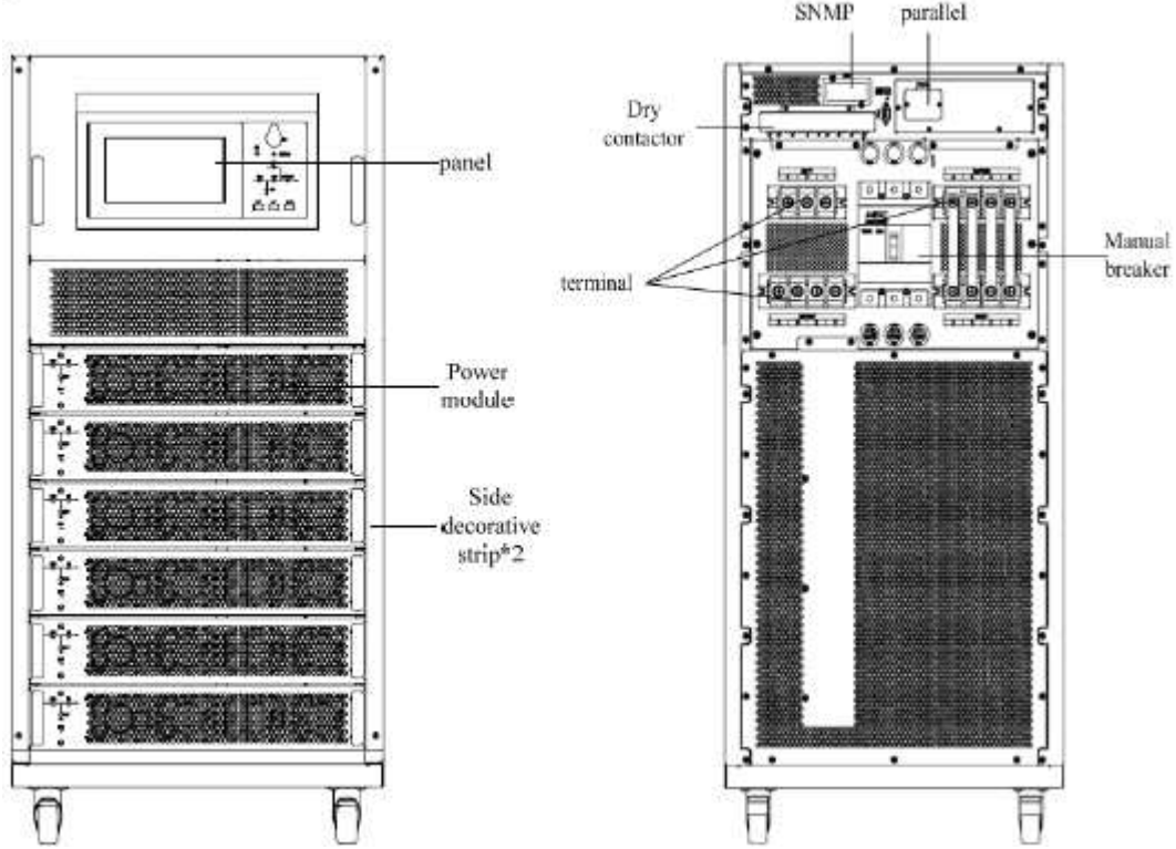
Şekil 4-3: 6 modül UPS Sistem, Kapısız Arkadan Görünüş
