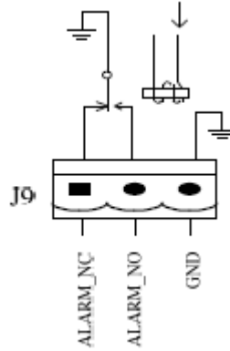
Şek.1- 12: Entegre uyarı kuru kontaktörü
