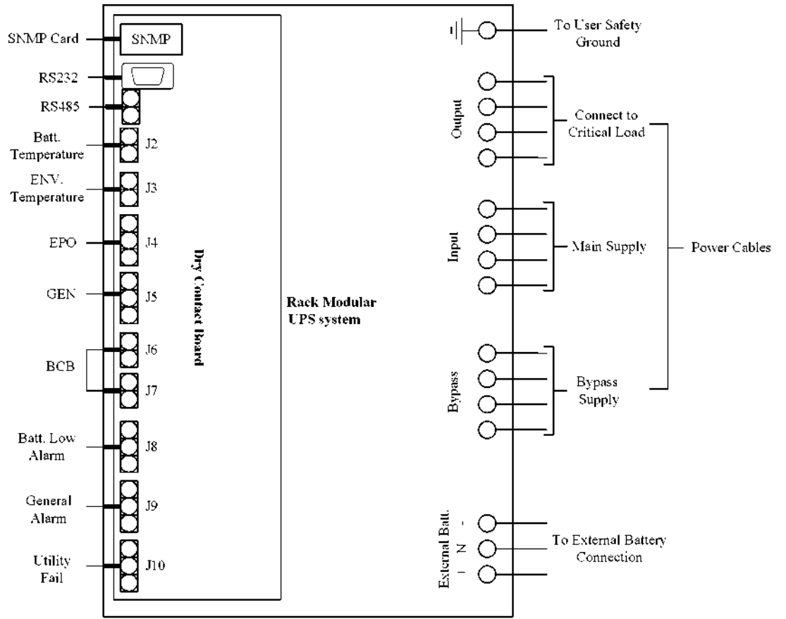
Şekil 4-1: Kablolama Şeması
