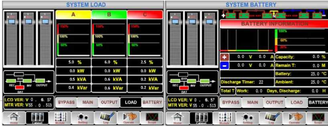
Şekil 7-6: yük ve akü bilgileri
