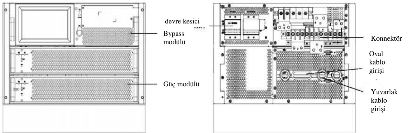
(d) 2 modüllü kabin
