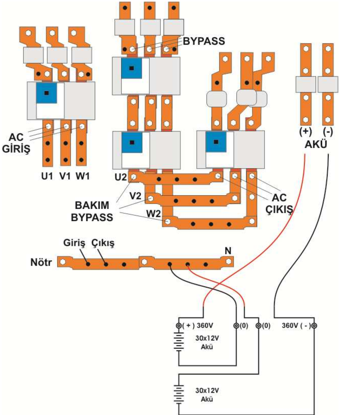
Şekil 2.2 DS3400T Kablo Bağlantısı
