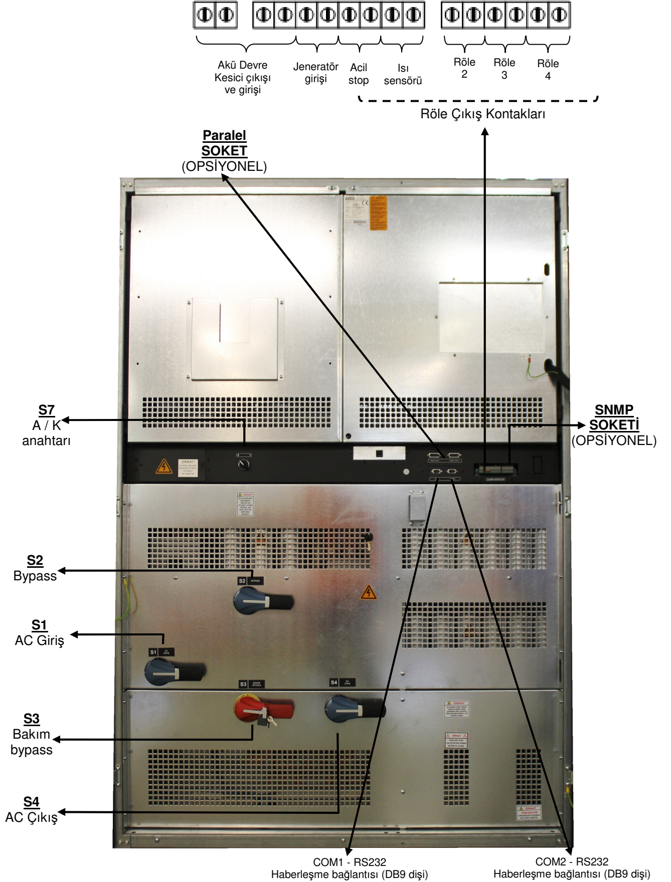
Şekil 1.3 400 kVA Sigorta ve Anahtar Düzeni, Arayüz Bağlantıları
