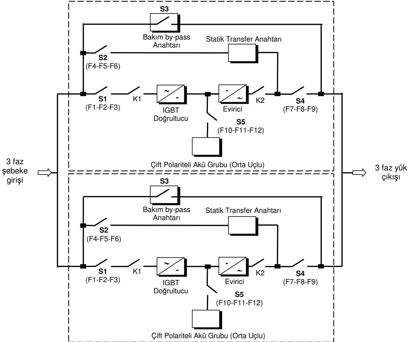
Figure 4.1 İki DS300T KGK'nın Paralel Bağlantısı
