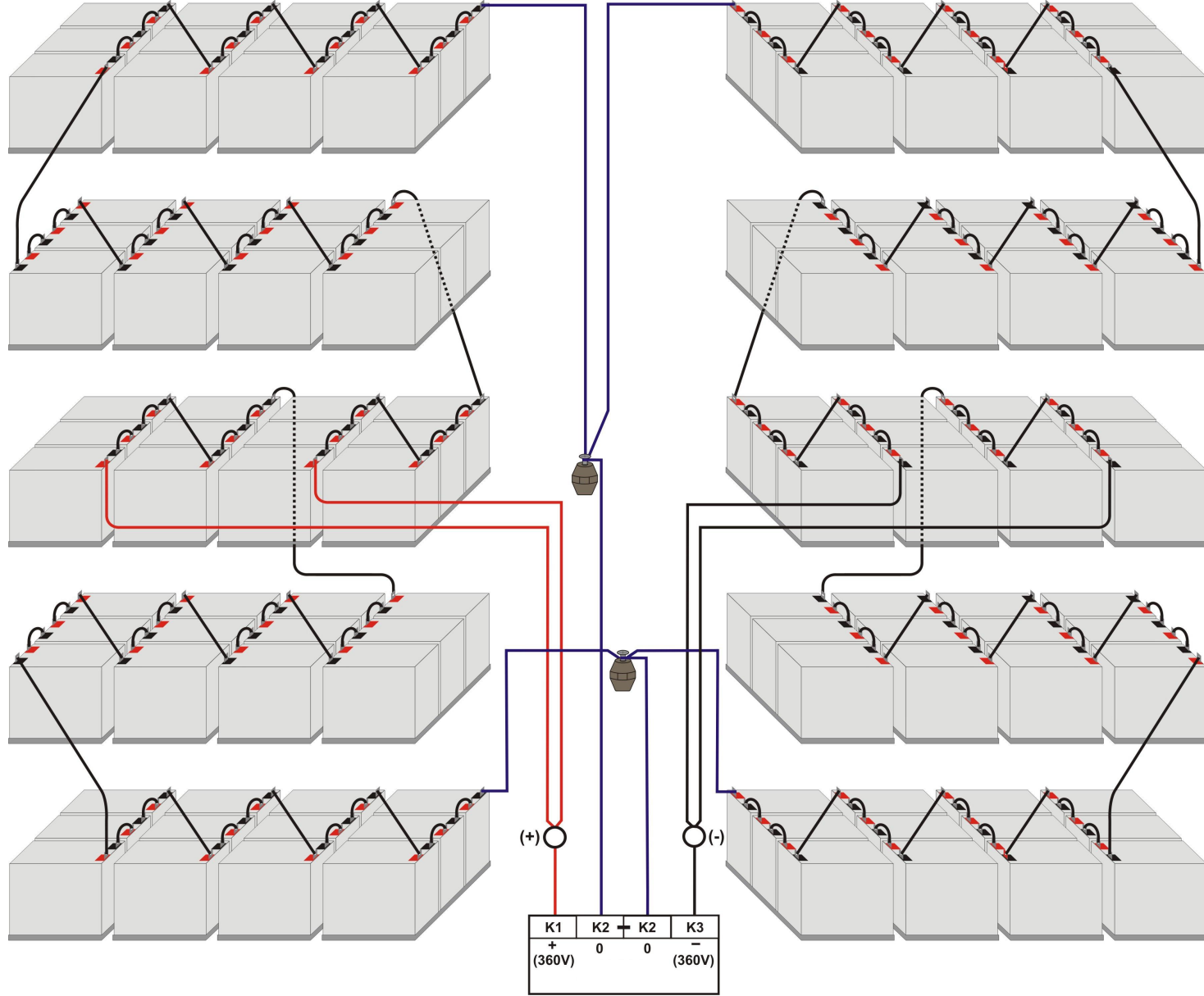
Şekil 2.5b DS300A, Dahili akü bağlantısı (2x60 pcs. 12V 7Ah) (orta uçlu iki grup akü paralel)
