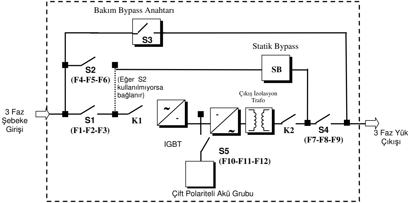
Şekil 1.1 DS300T Serisi UPS Blok Şeması
