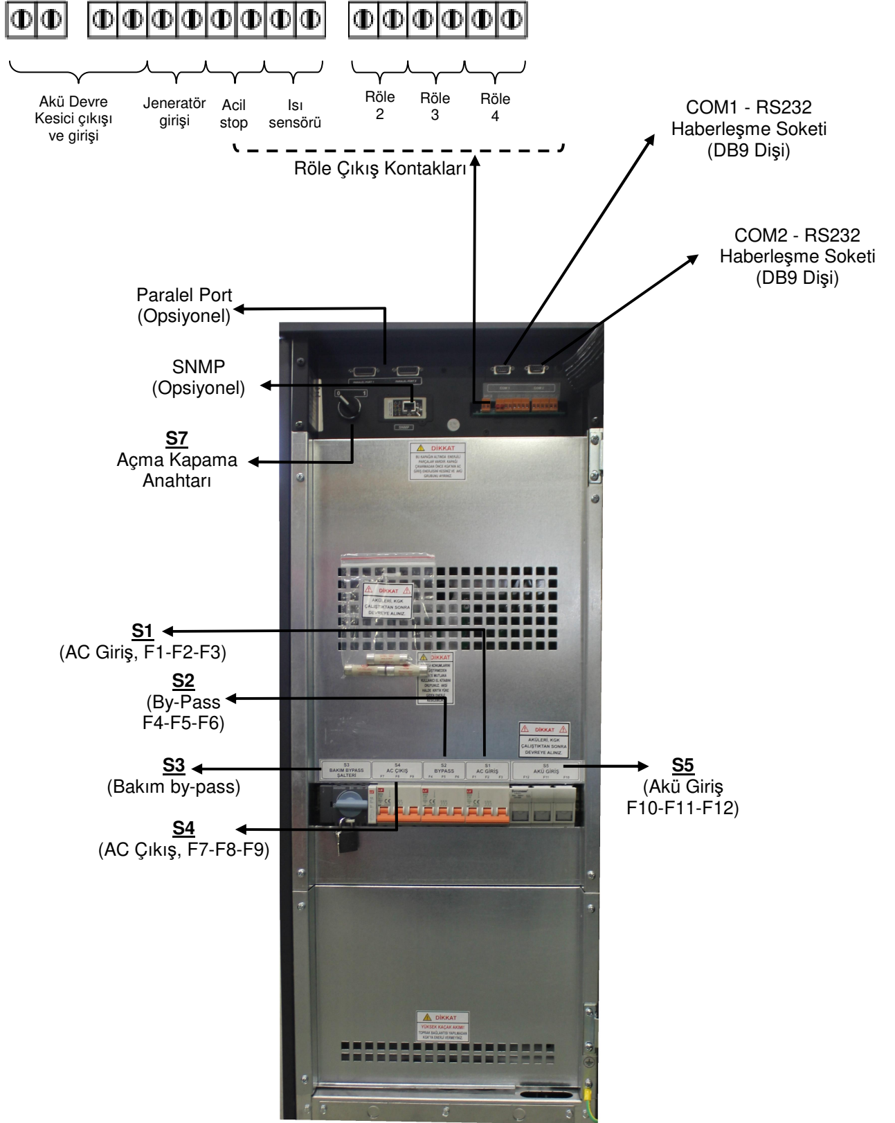
Şekil 1.3 a 10-15-20-30 kVA Sigorta ve Anahtar düzeni
