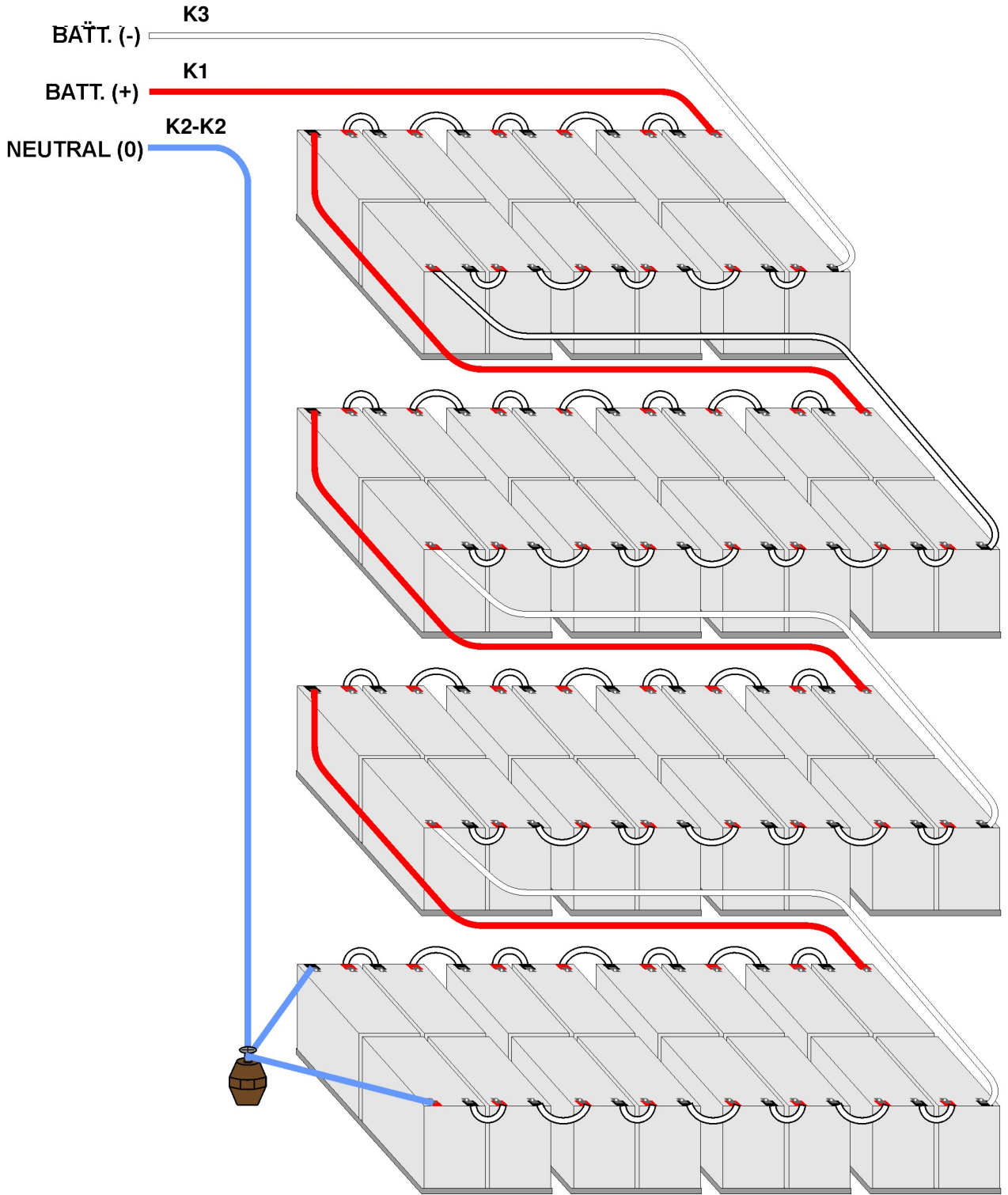
Şekil 2.5a DS300HA Serisi 10-15-20-30 KVA Dahili Akü bağlantıları (2x30=60x12V 7Ah)
