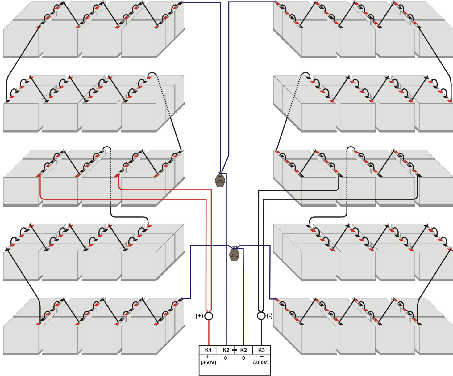
Şekil 2.5b DS300HA, Dahili akü bağlantısı (2x60 pcs. 12V 7Ah) (orta uçlu iki grup akü paralel)
