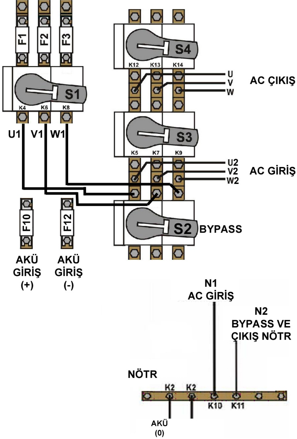
Şekil 2.2 120kVA Kablo Bağlantısı
