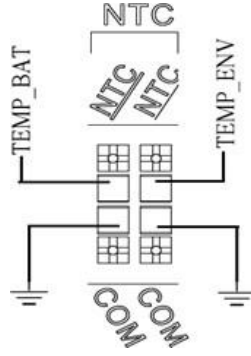
Şekil 3-14 Sıcaklık algılama için NTC
