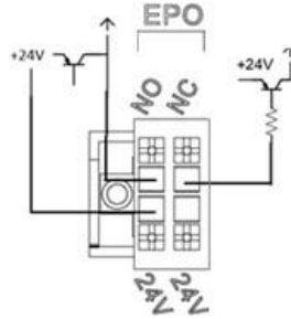
Şekil 3-15 Uzaktan EPO için giriş port şeması
