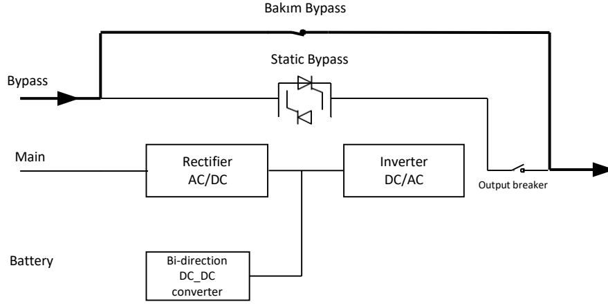
Şekil 2-6 Bakım modunda UPS kavramsal şeması
