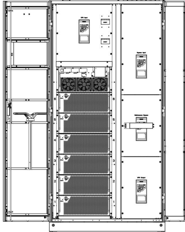
Şekil 2-8 UPS Kabini önden görünümü
