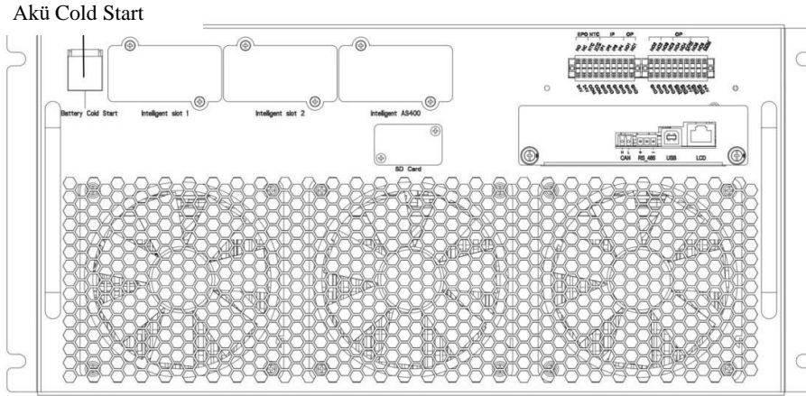
Şekil 5-1 Akü cold start düğmesinin kabin üzerindeki konumu
