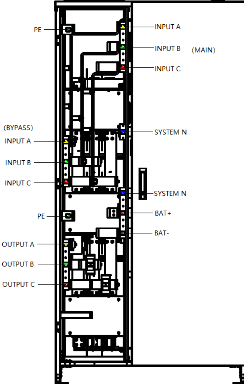
Şekil 3-11 Bağlantı terminalleri
