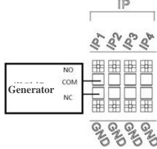
Şekil 3-16 Durum arayüzü ve jeneratör bağlantısı şeması
