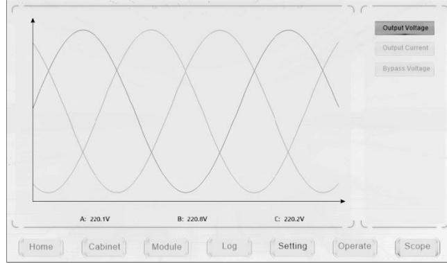
Şekil 4-11 Ölçüm Menüsü
