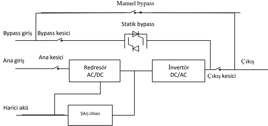
Şekil 2-1 UPS sistem şeması
