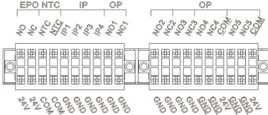
Şekil 3-13 Kuru Kontak Arayüzü Tablo 3-5 Port Fonksiyonları
