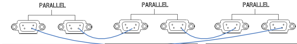
Şekil 5-7 Paralel Bağlantı
