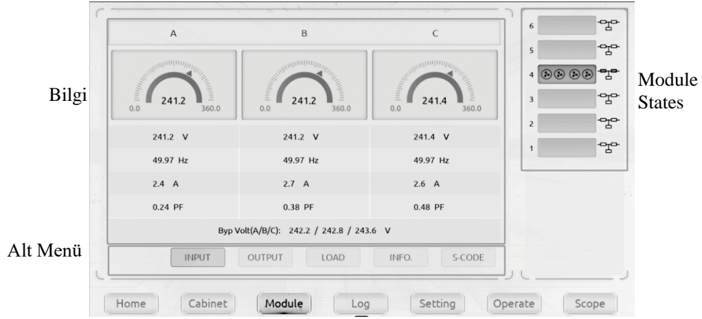
Şekil 4-6 Güç Modülü
