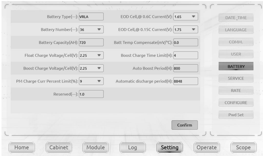
Şekil 5-3 Akü otomatik deşarj için süre ayarı
