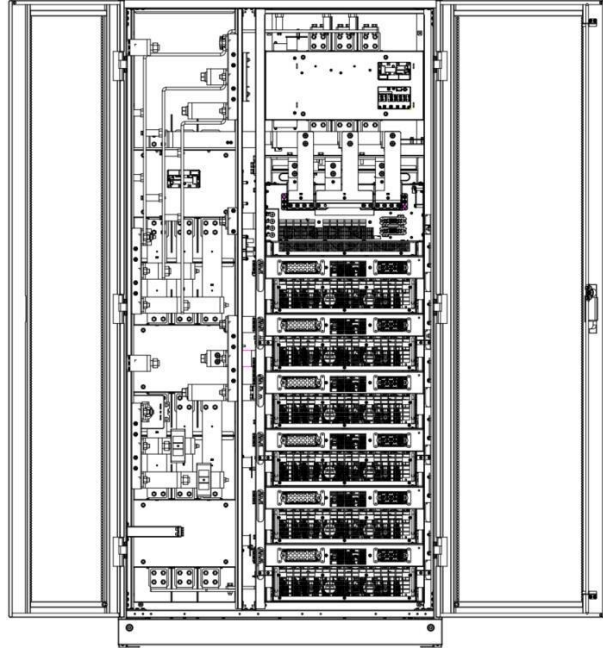
Şekil 2-9 UPS Kabini arka görünümü
