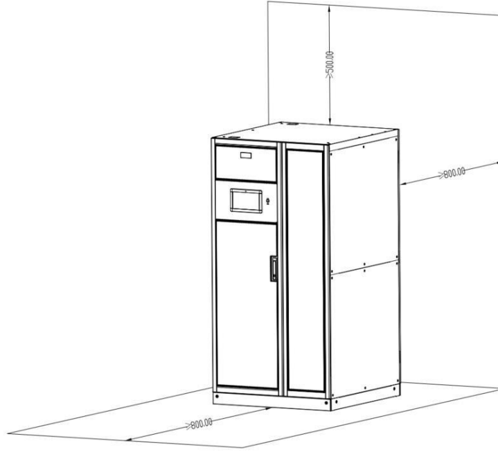
Şekil 3-2 Ayrılmış Kabin Alanı (birim: mm)
