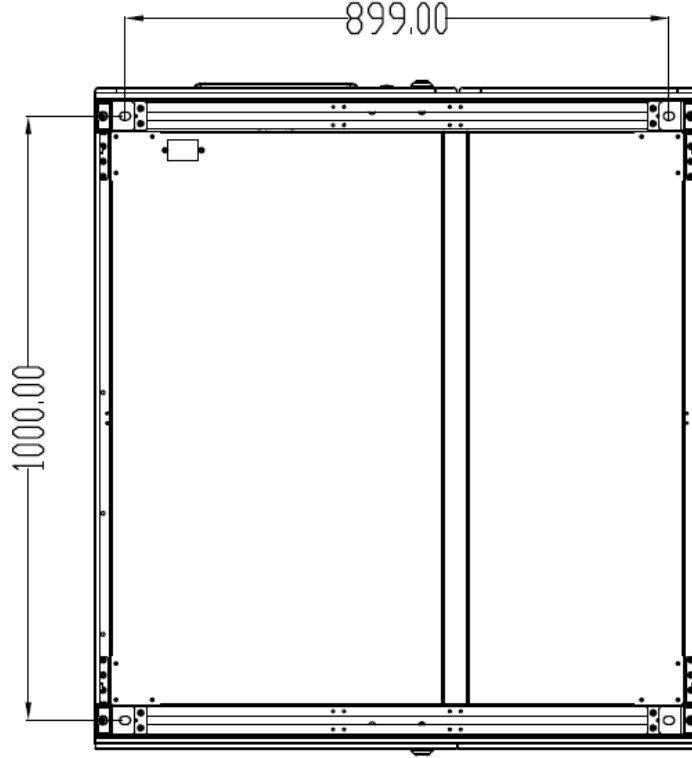
Şekil 3-6 Destekleyici yapı (Altan görünüm)
