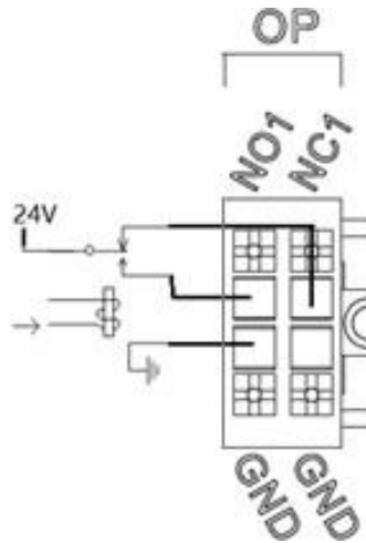
Şekil 3-18 Akü uyarısı kuru kontak arayüz şeması
