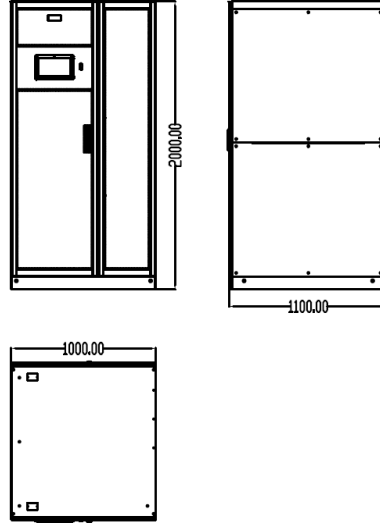
Şekil 3-1 Kabin Boyutları (birim: mm)
