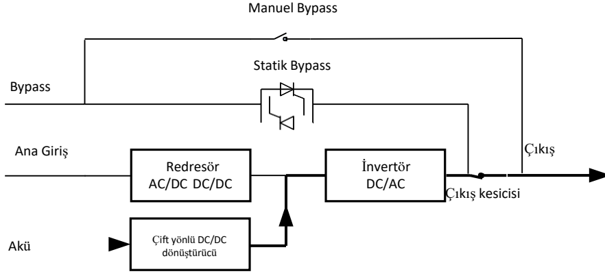
Şekil 2-4 Akü Modunda UPS Kavramsal Şeması
