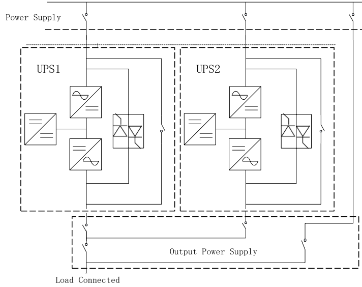
Şekil 5-5 Paralel şema
