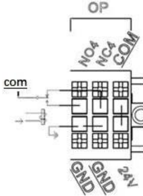
Şekil 3-19 Şebeke arızası uyarısı kuru kontak arayüz şeması
