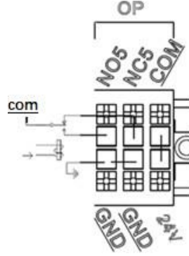
Şekil 3-20 Aşırı Yük Alarm Girişi Kuru Kontak Arayüzü Şeması
