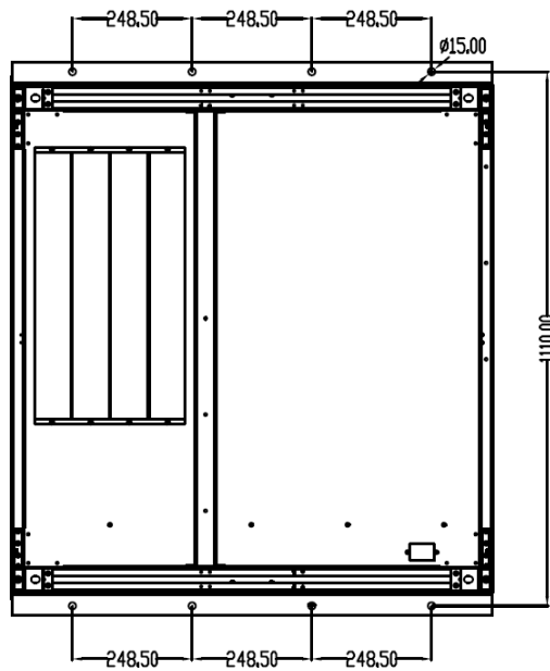
Şekil 3-8 Sismik sabit cihazın boyutlu çizimleri
