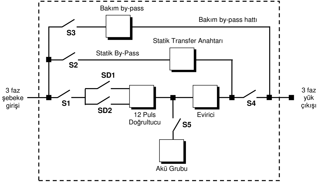
Şekil 1-1 Blok Diagram
