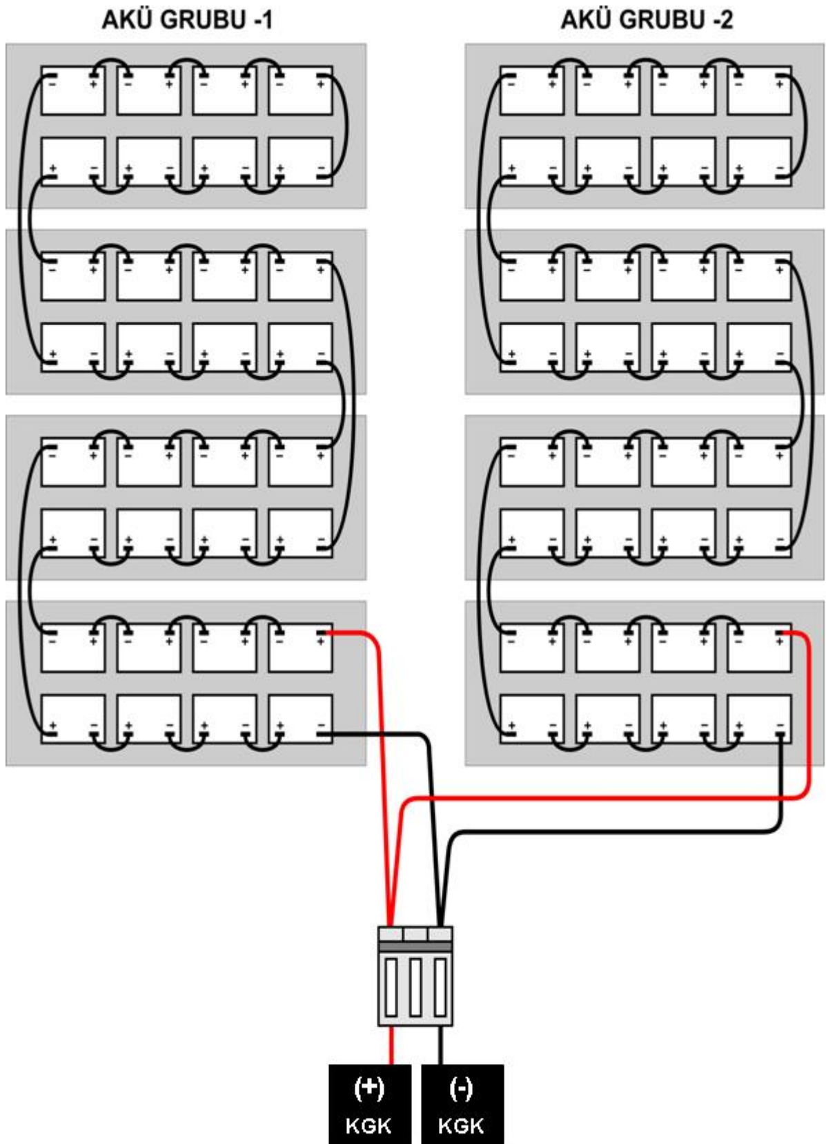
Şekil 5-3-b 250 kVA KGK Akü Grubu Bağlantısı
