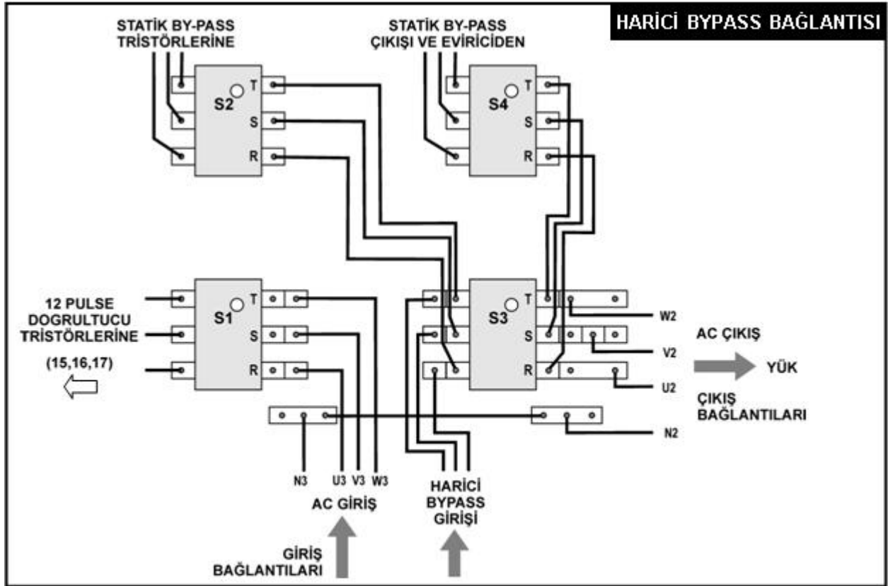
Şekil 5-2-b 250-300 kVA KGG Güç Bağlantısı
