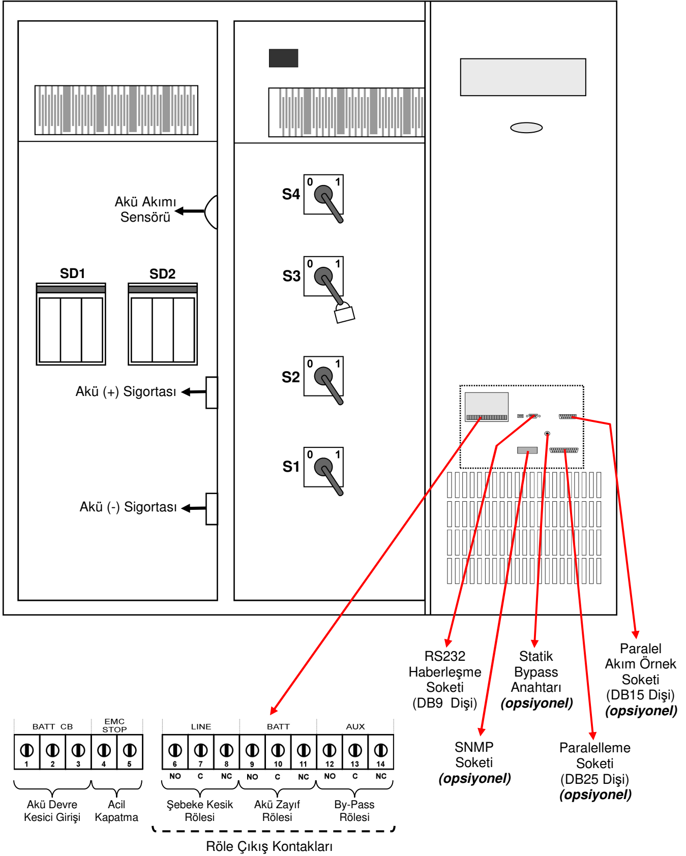
Şekil 1-3-a 200 kVA sigorta ve anahtar düzeni
