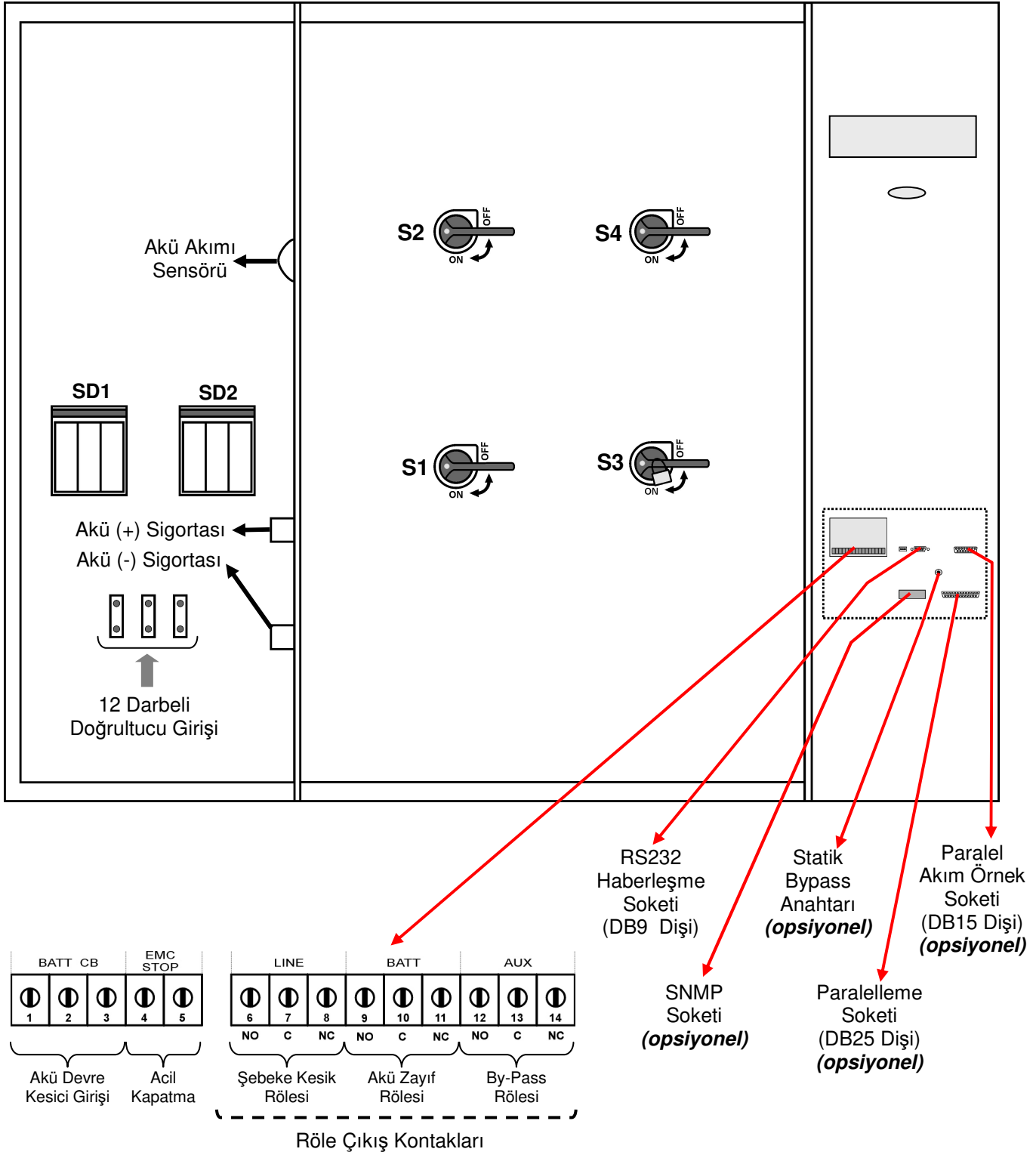
Şekil 1-3-b 250-300 kVA sigorta ve anahtar düzeni
