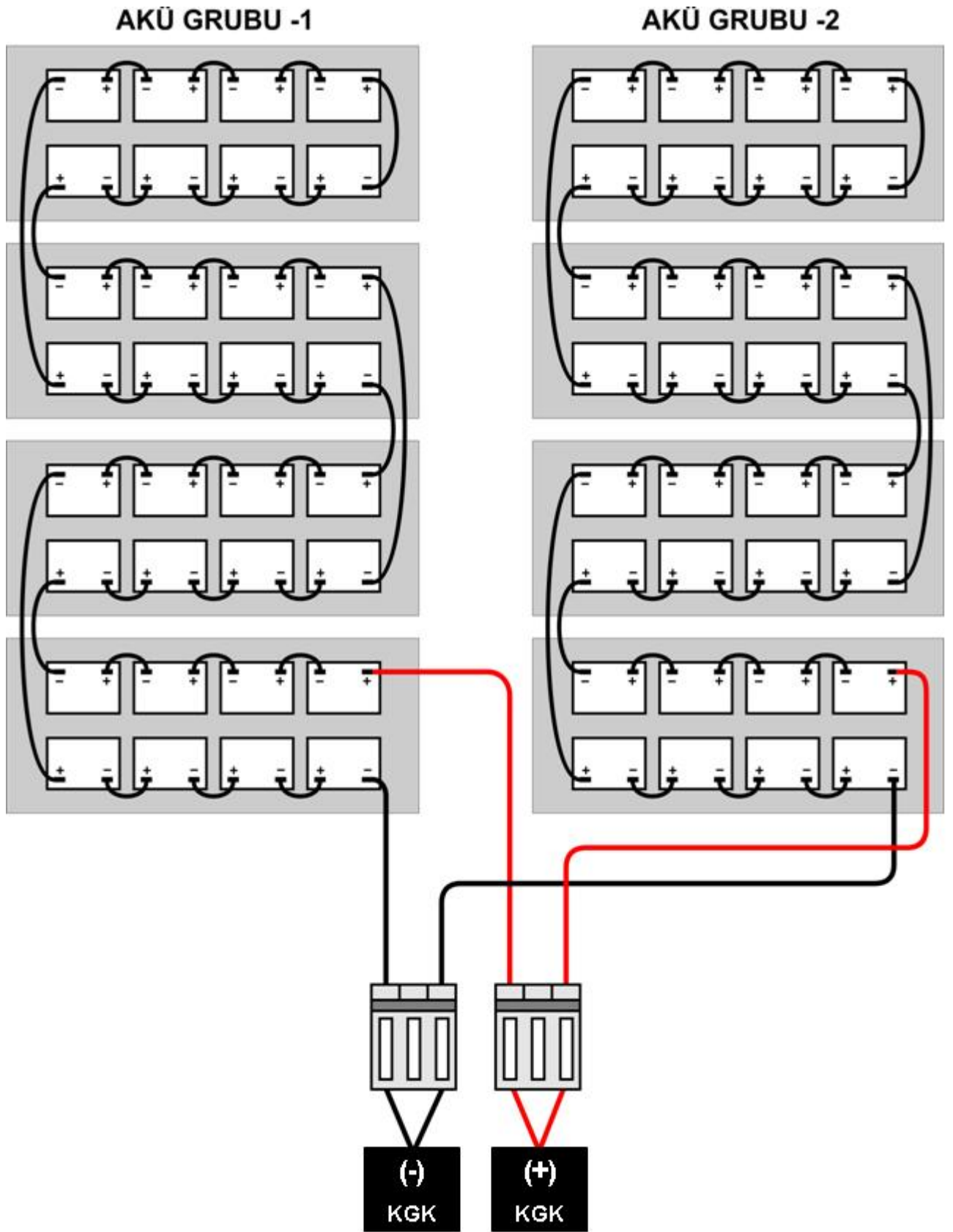
Şekil 5-3-c 300 kVA KGC Akü Grubu Bağlantısı
