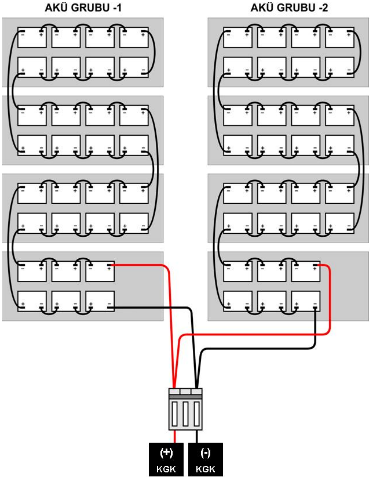
Şekil 5-3-a 200 kVA KVK Akü Grubu Bağlantısı
