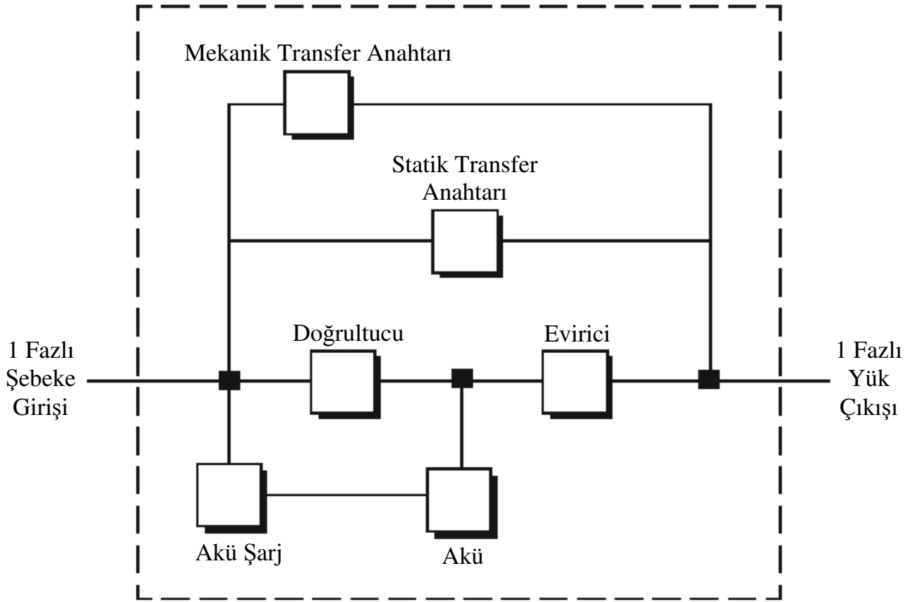
Şekil 1.1 KKGK Blok Şeması
