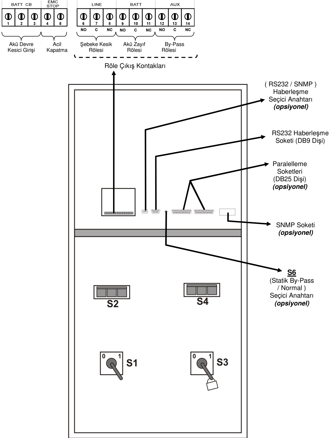
Şekil 1-3-a 40-45-50-60 kVA sigorta ve anahtar düzeni
