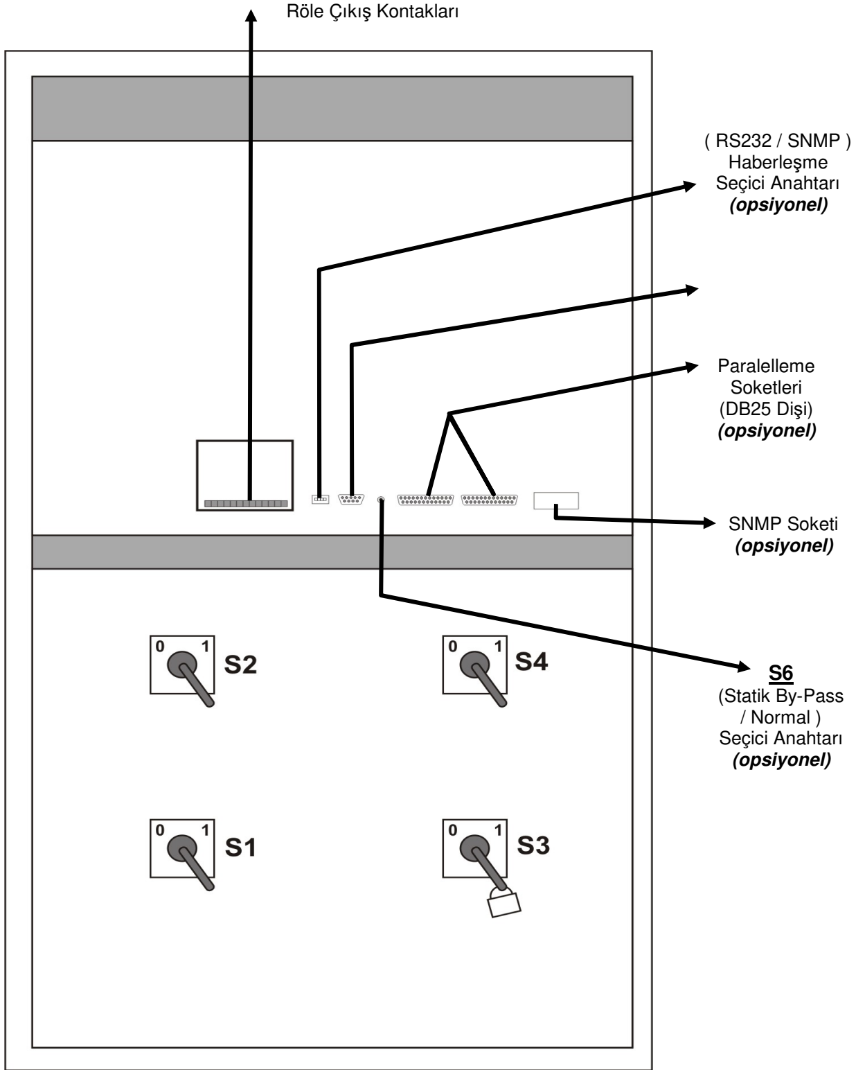
Şekil 1-3-b 80 kVA sigorta ve anahtar düzeni
