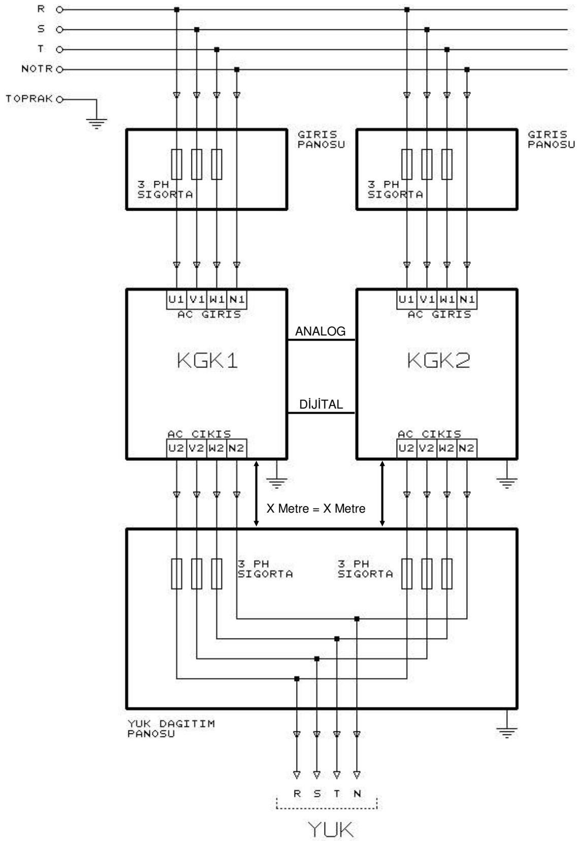
Şekil 5-2 Paralel KGGK Sistem Şeması
