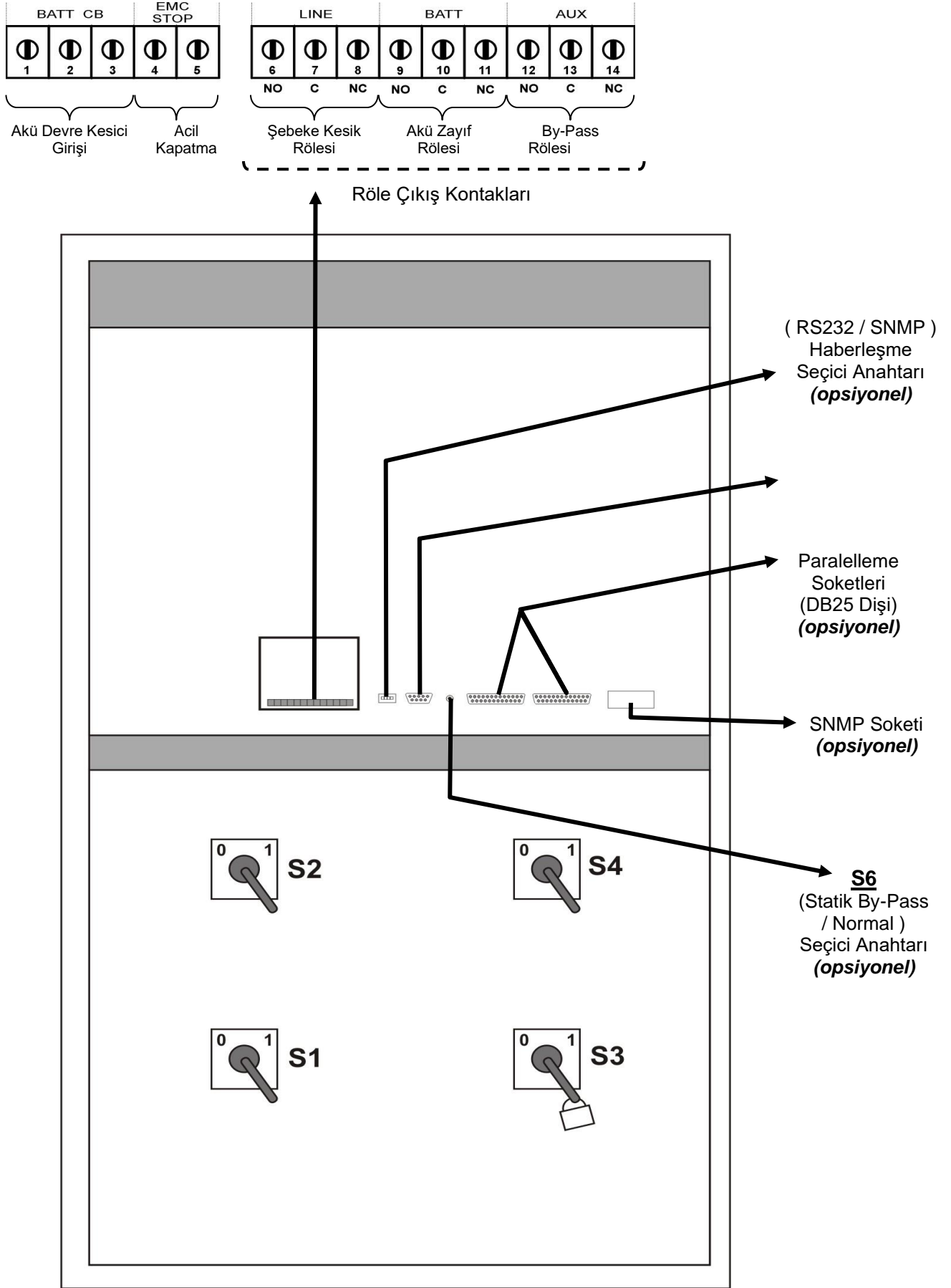
Şekil 1-3-b 80 kVA sigorta ve anahtar düzeni
