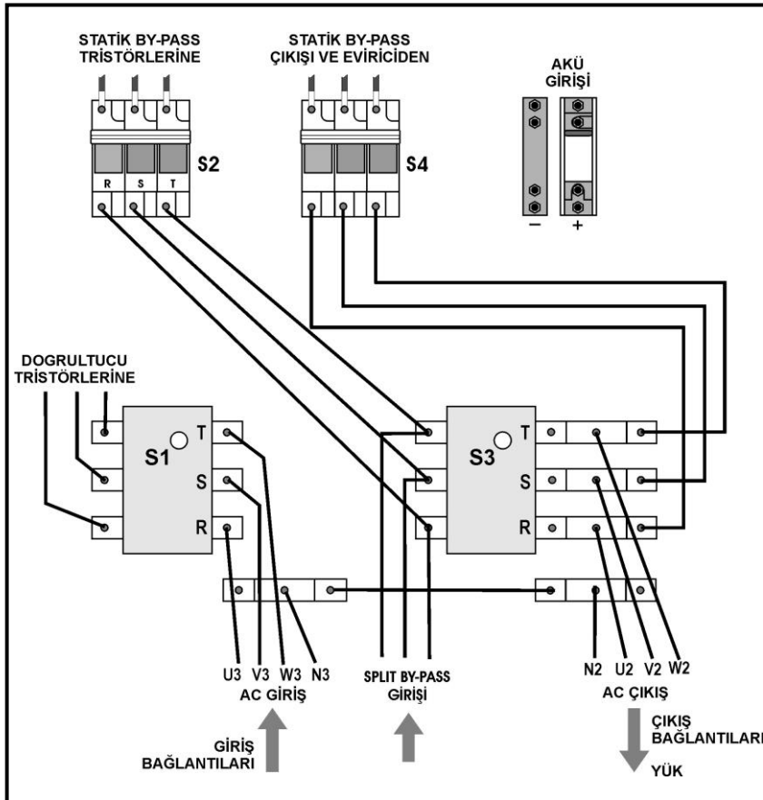
Şekil 3-2-a 40-45-50-60 kVA KGK Güç Bağlantısı
