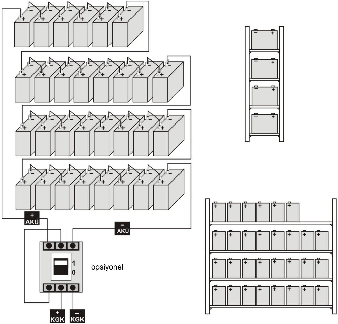
Şekil 3-3-b KGK Akü Grubu Bağlantısı (Opsiyonel)
