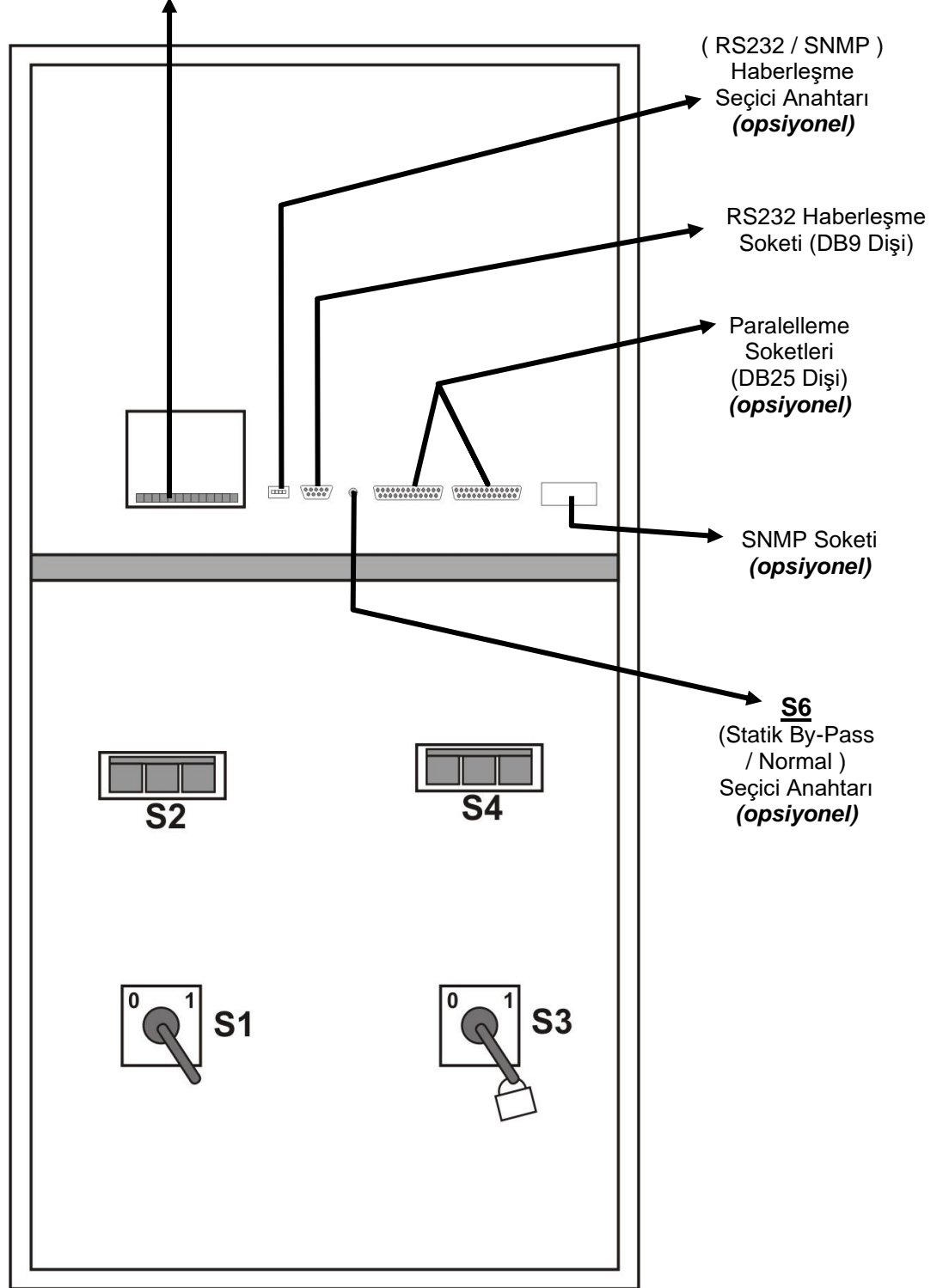
Şekil 1-3-a 40-45-50-60 kVA sigorta ve anahtar düzeni
