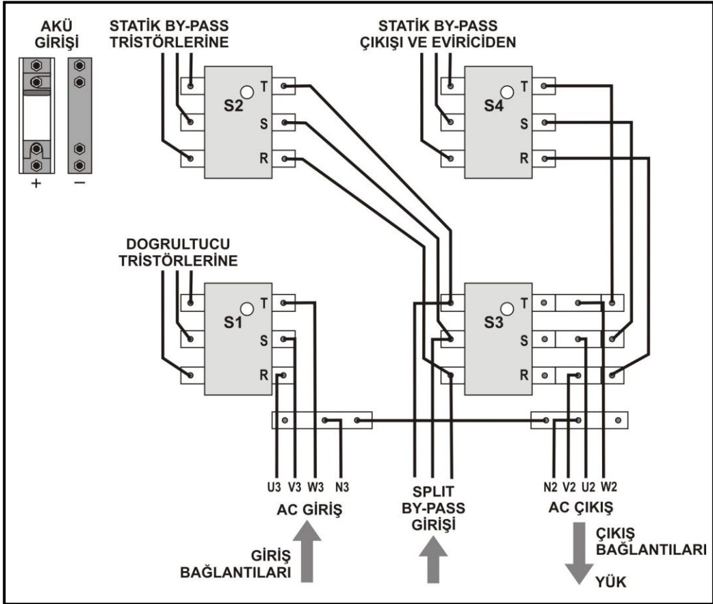
Şekil 3-2-b 80 kVA KVK Güç Bağlantısı
