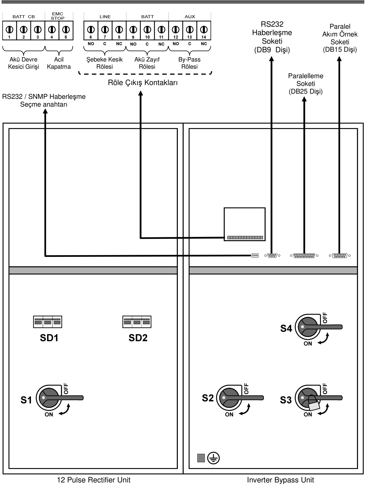
Şekil 1-3 80 kVA sigorta ve anahtar düzeni
