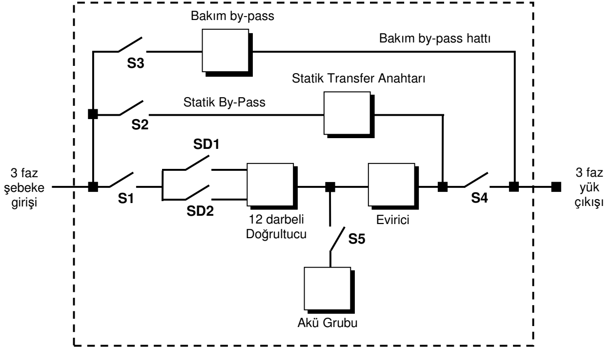
Şekil 1-1 Blok Diagram
