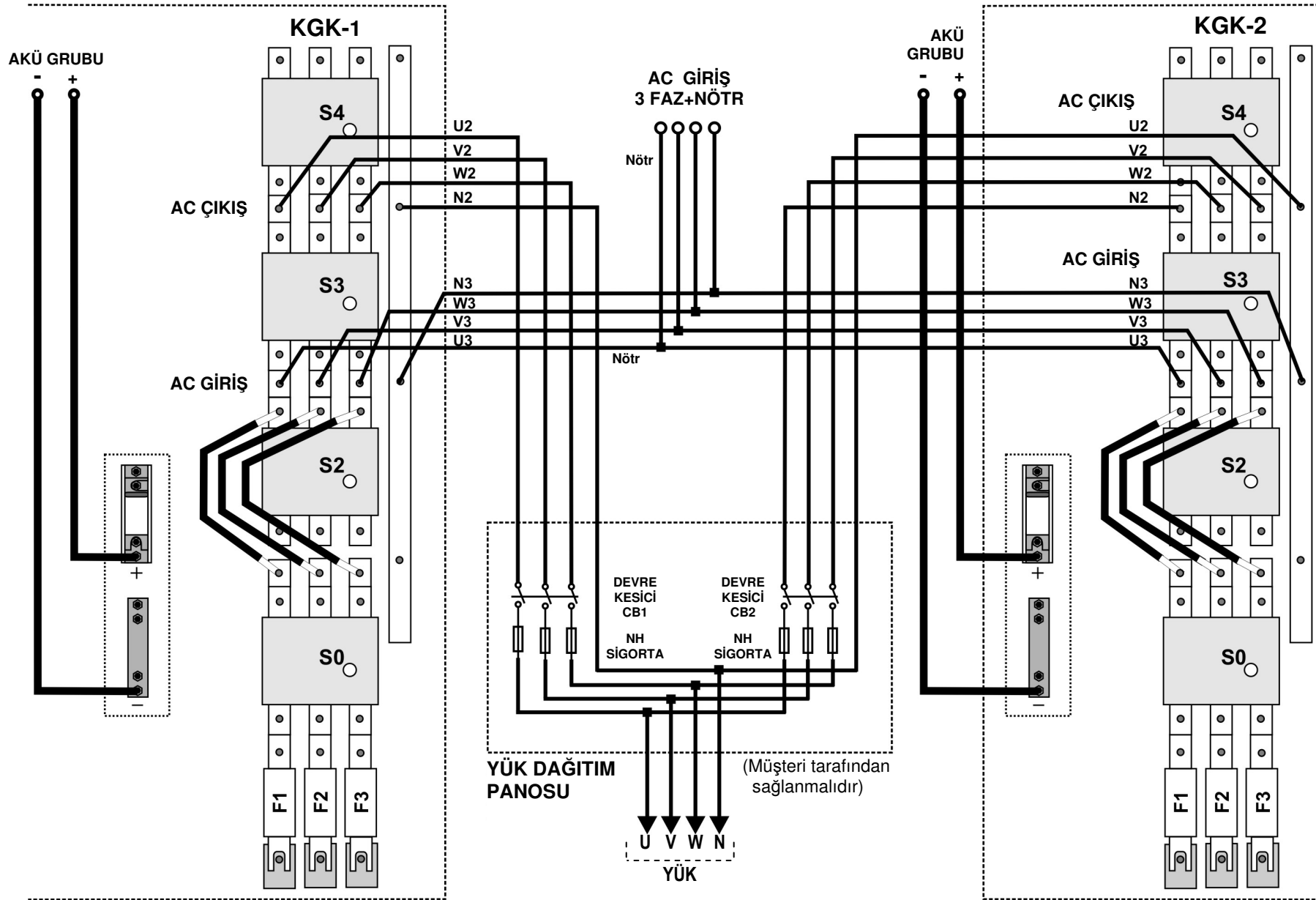
Şekil 5-3 PARALEL ÇALIŞTIRMA İÇİN İKİ KGK'NİN GÜÇ BAĞLANTILARI (80-100 kVA)
