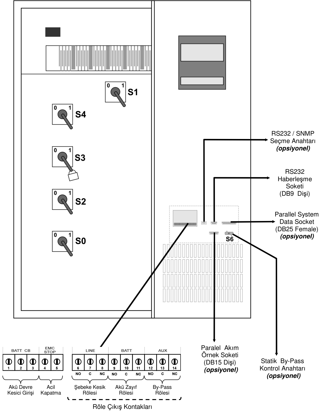
Şekil1-3 80-100 kVA sigorta ve anahtar düzeni
