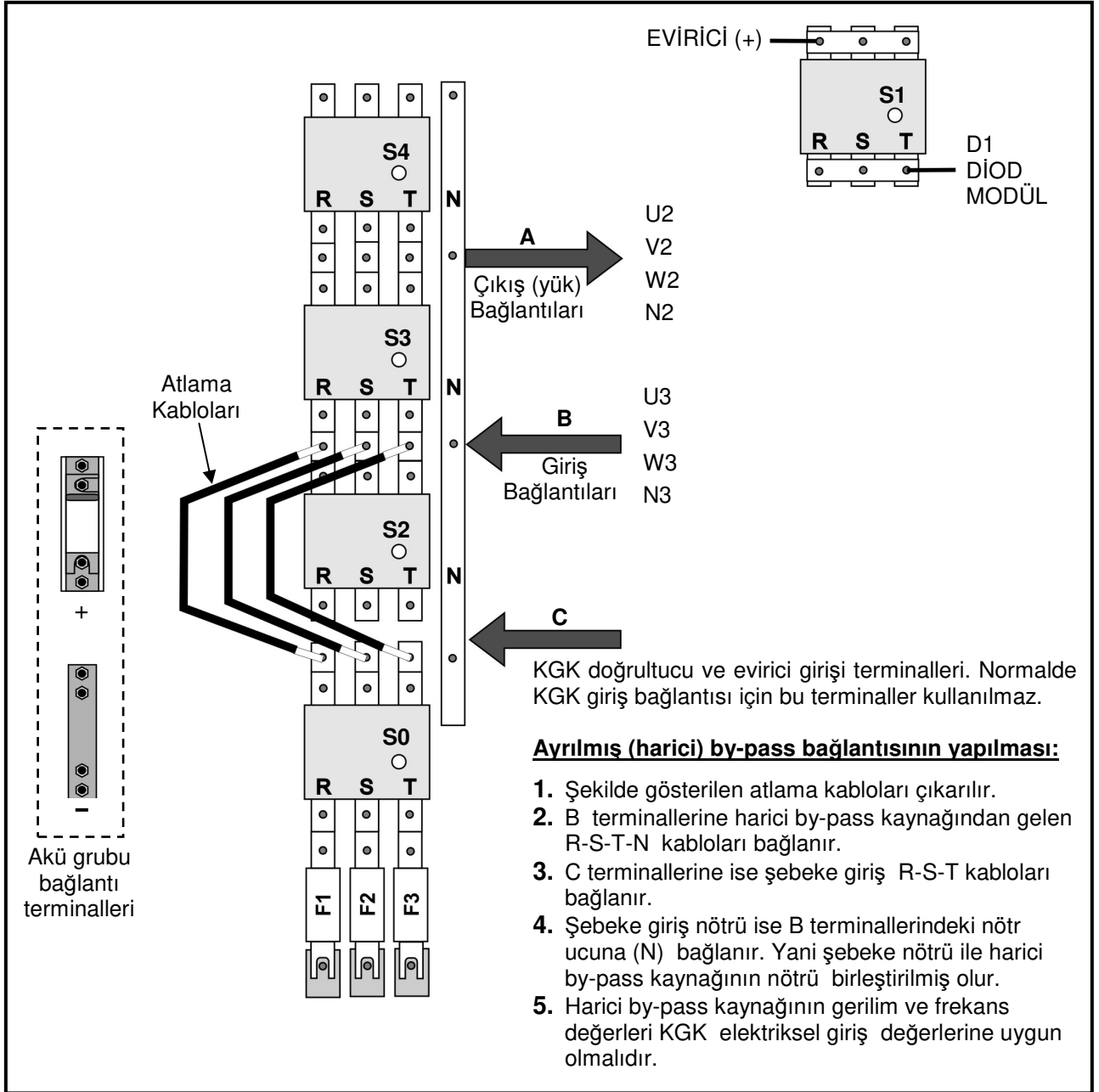
Şekil 5-2 80-100 kVA KGK Güç Bağlantısı
