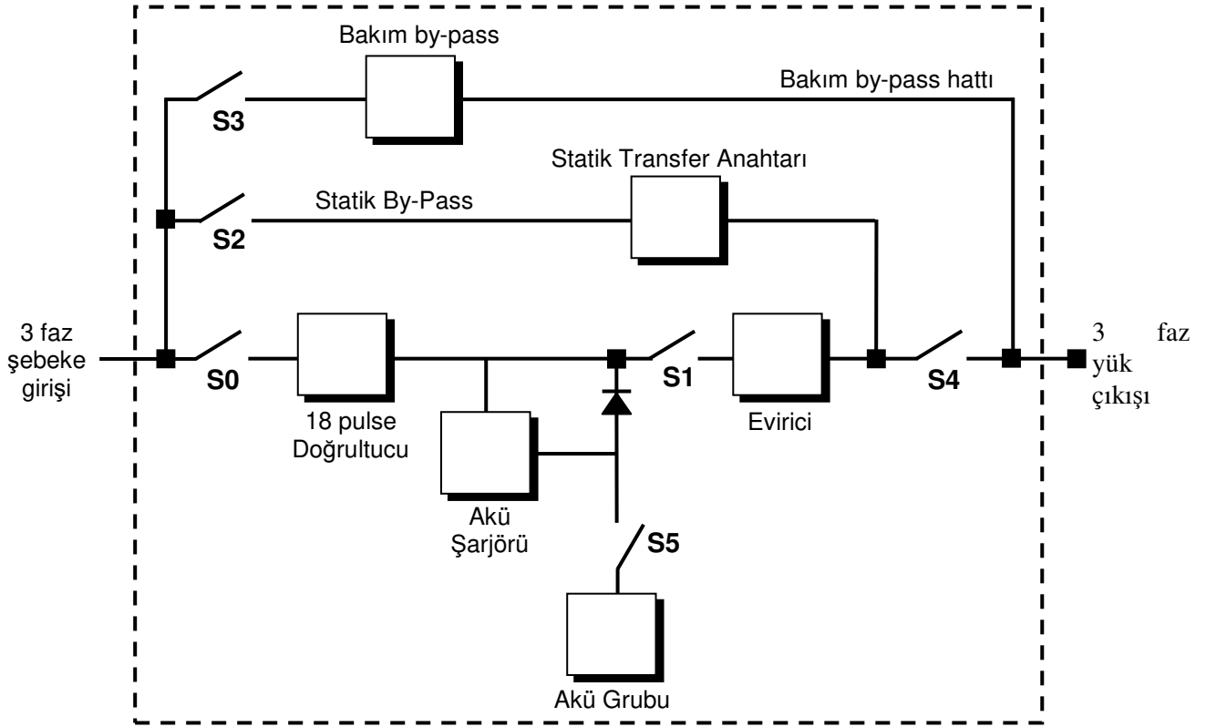
Şekil 1-1 Blok Diagram
