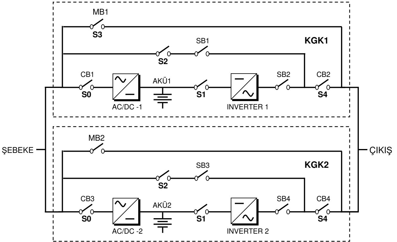
Şekil 3-1 Paralel bağlı 2 KGK
