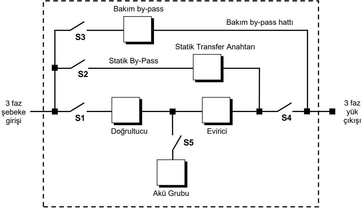
Şekil 1-1 Blok Diagram
