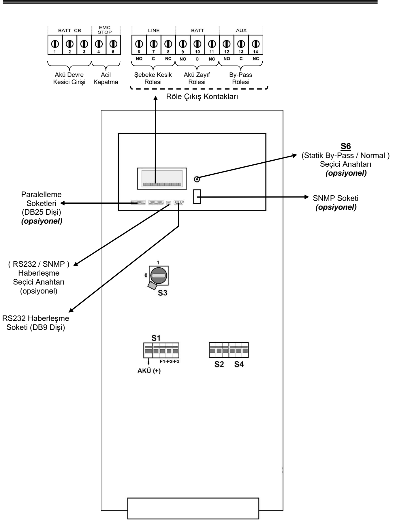
Şekil 1-3-c 30 kVA sigorta ve anahtar düzeni
