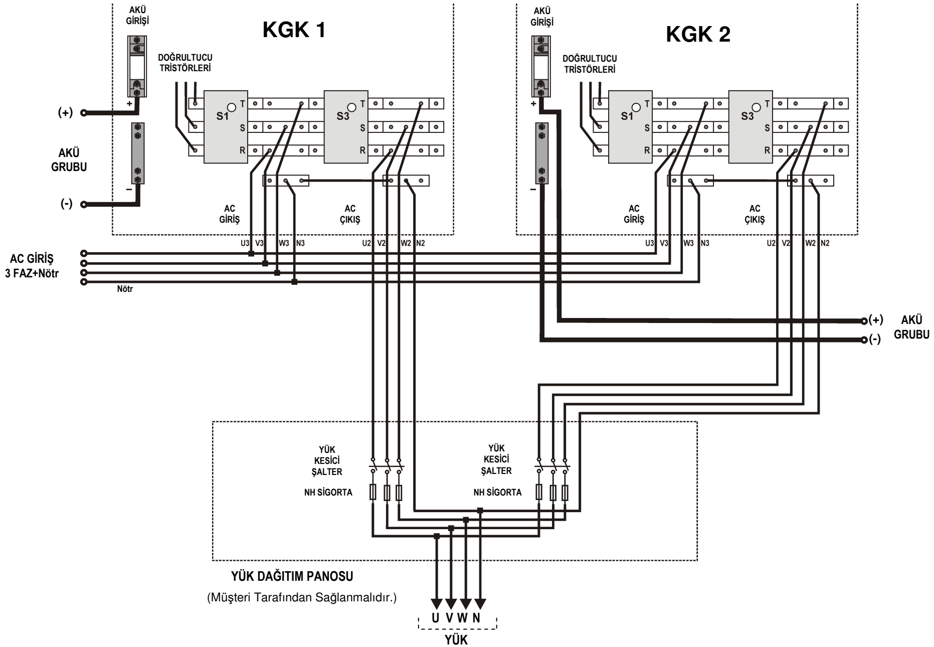
Şekil 3-3 PARALEL ÇALIŞTIRMA İÇİN İKİ KGK'NIN GÜÇ BAĞLANTILARI (250-300kVA)
