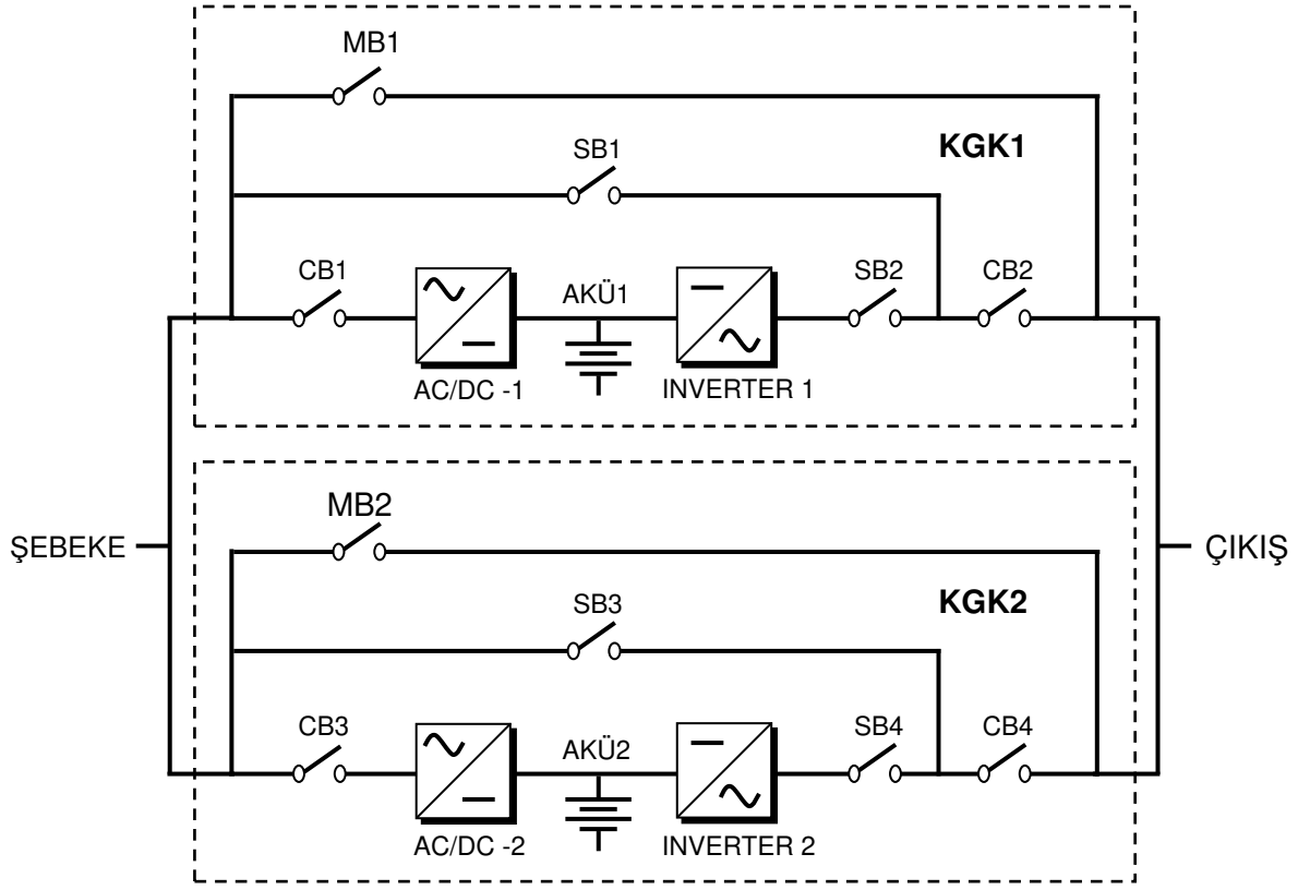
Şekil 5-1 Paralel bağlı 2 KGK
