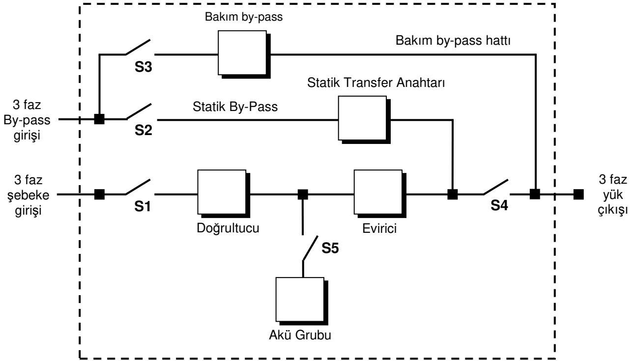
Şekil 1-1 Blok Diagram
