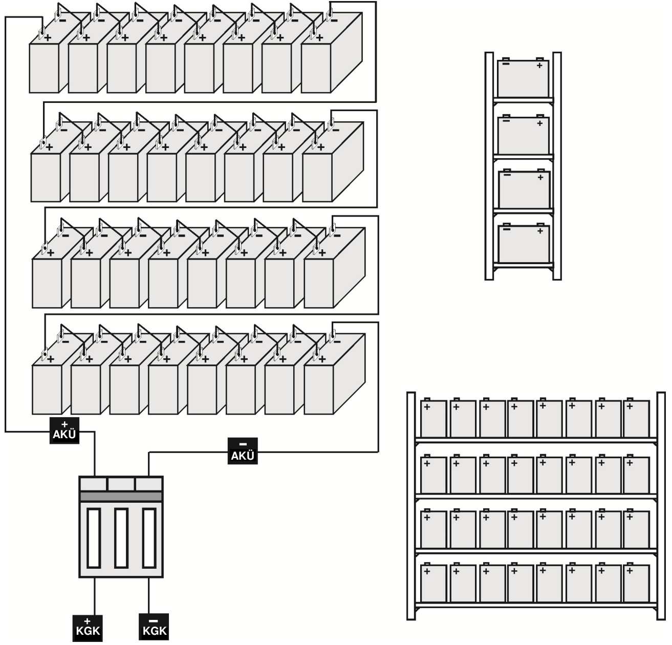
Şekil 3-4 KGK Akü Grubu Bağlantıları
