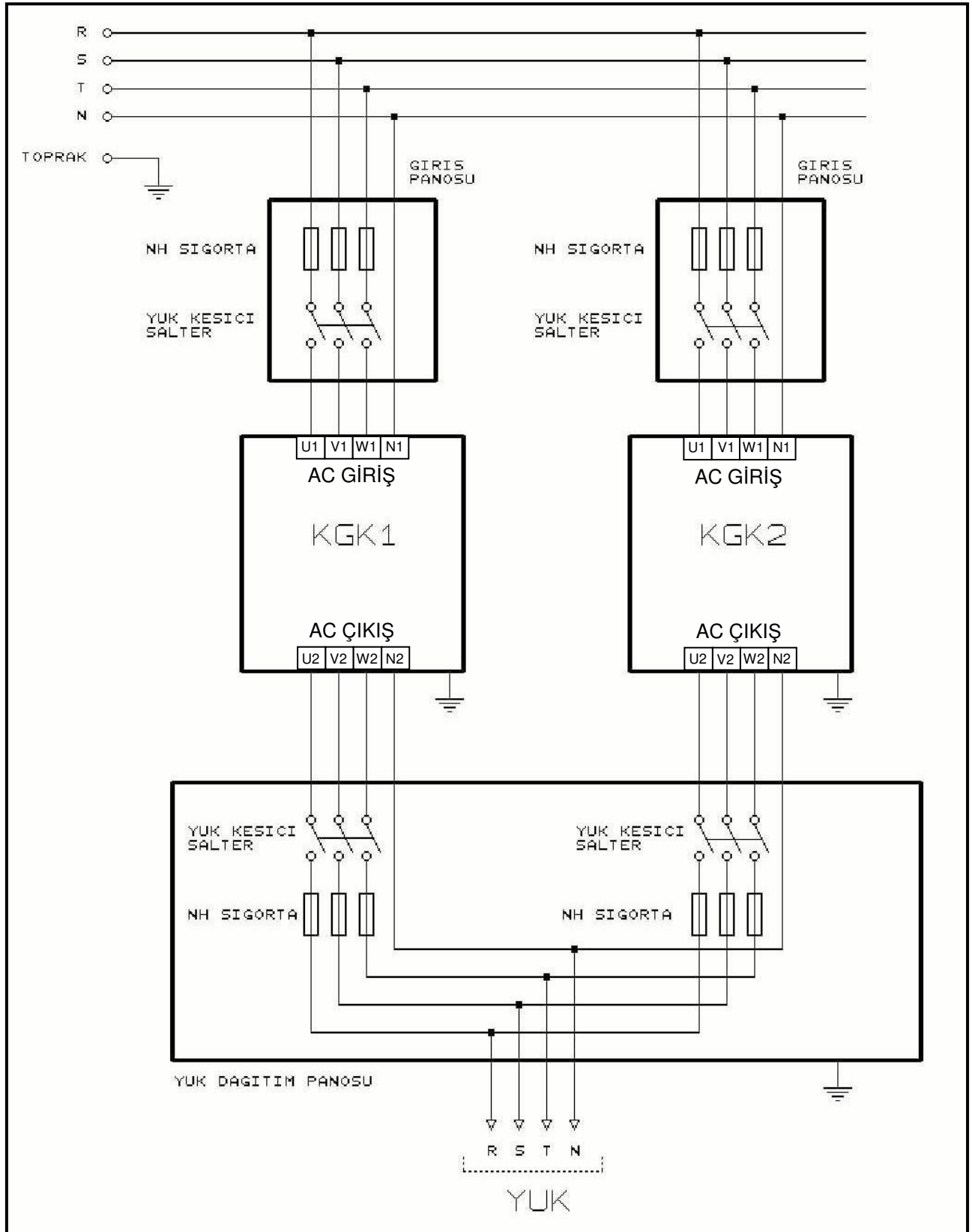
Şekil 5-2 Paralel KGK Sistem Şeması
