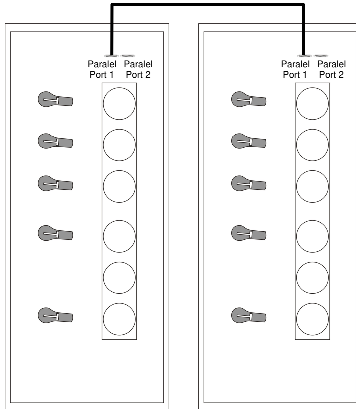
Şekil 4.2.a İki KGK'nın Paralel Bağlantısı
