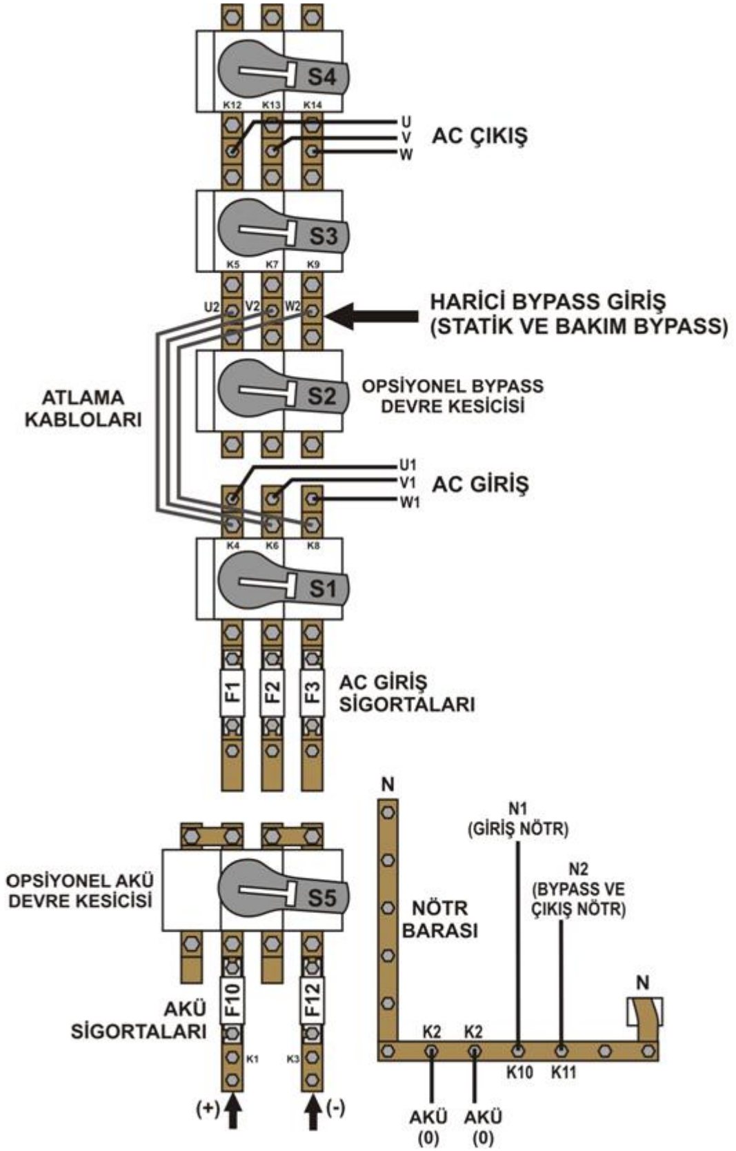
Şekil 2.2.a 100-120-160-200 kVA Giriş/Çıkış Kablo Bağlantıları (Bypass ve Akü Devre Kesicisi varsa (S2 ve S5) )
