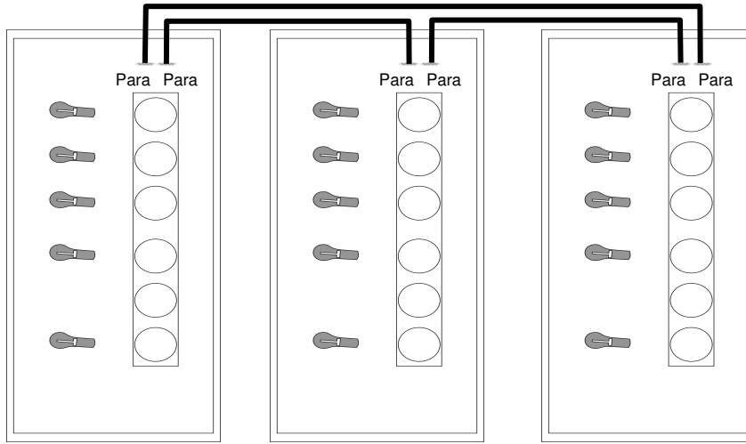
Şekil 4.2.b Üç KGK'nın Paralel ağılantısı
