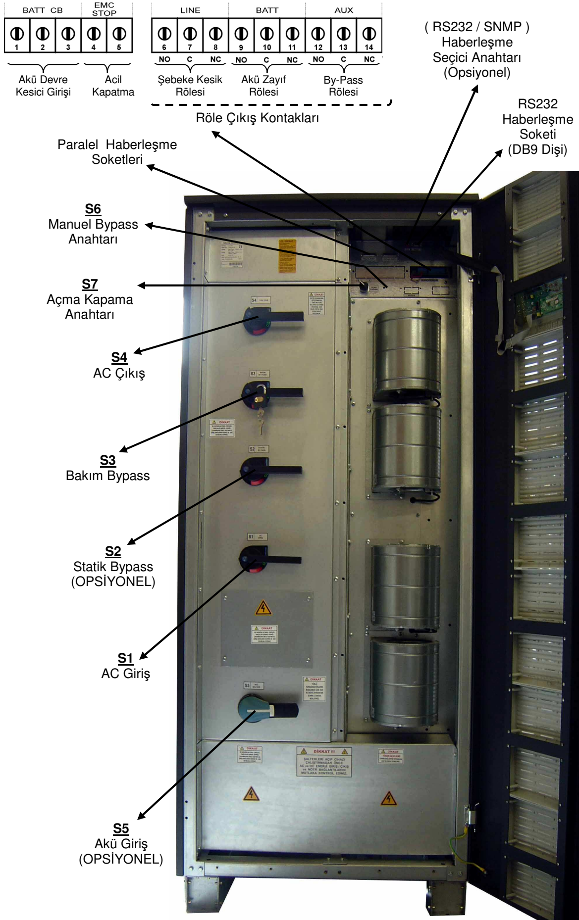
Şekil 1.3 100-120-160-200 kVA Sigorta ve Anahtar düzeni
