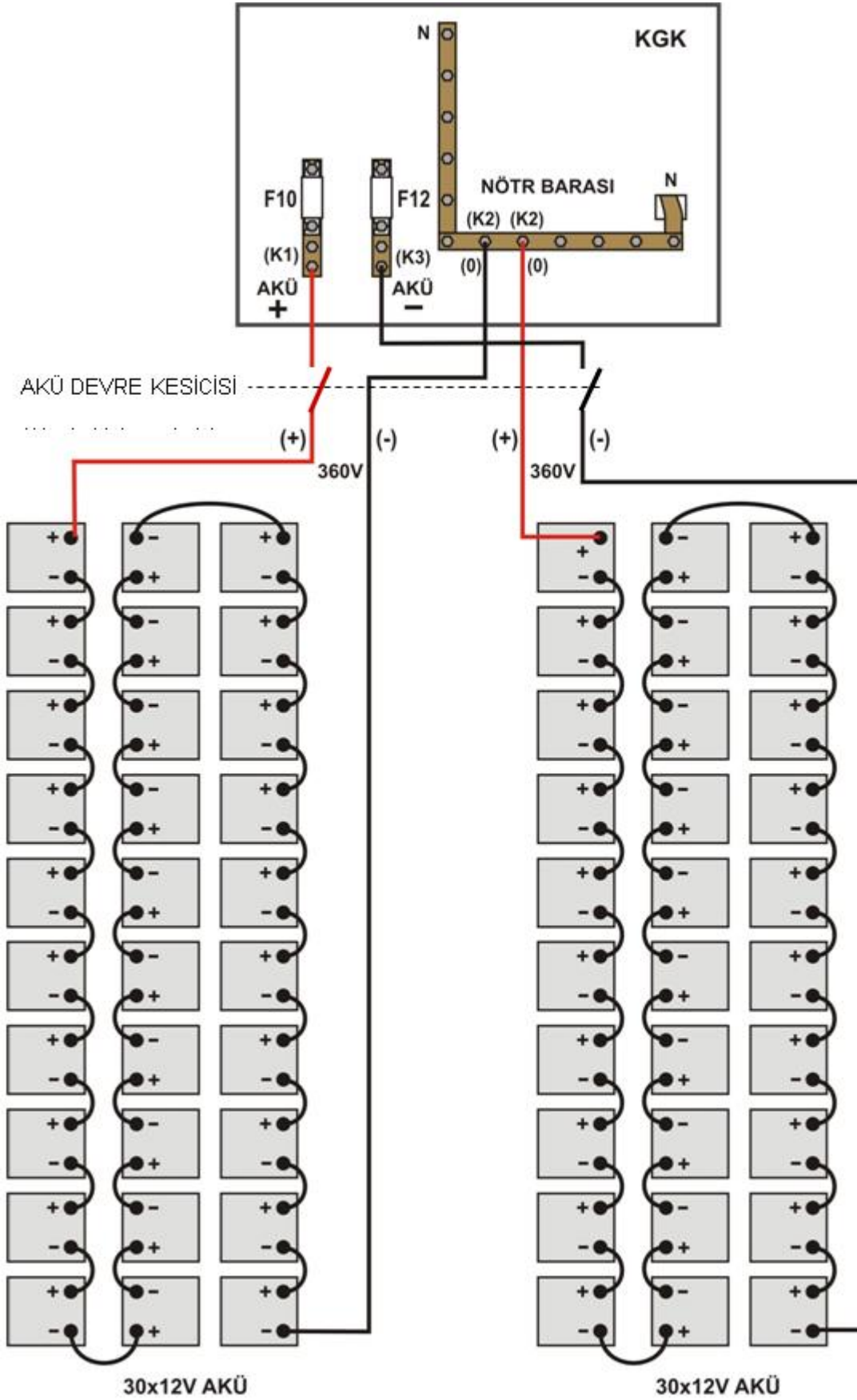
Şekil 2.4 CYCLONE 300P 100-120-160-200 KVA Aku bağlantıları
