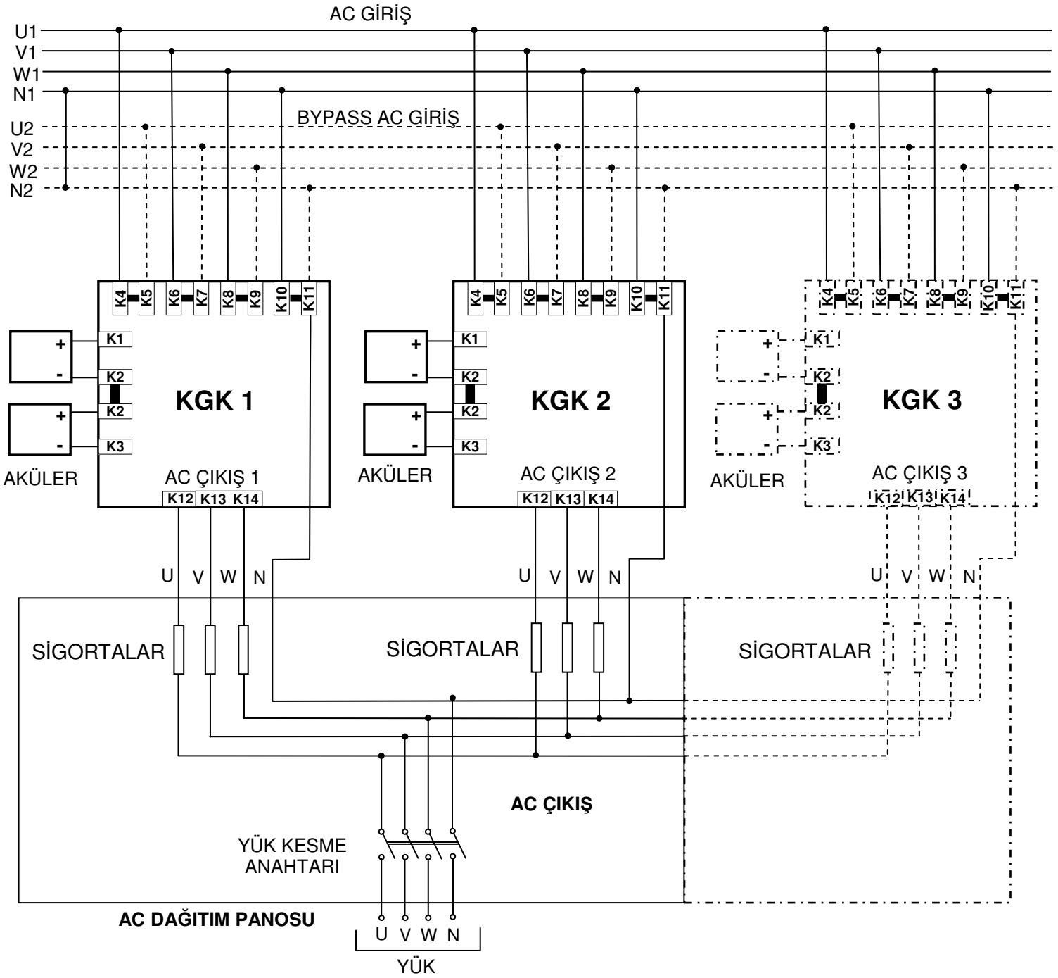
Şekil 4.3 CYCLONE 300P Serisi Paralel KGK Güç Bağlantıları
