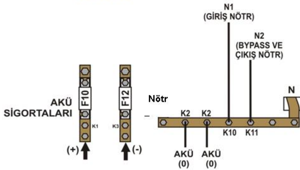
Şekil 2.2.b 100-120-160-200 kVA Giriş/Çıkış Kablo Bağlantıları ( Bypass ve Akü Devre Kesicisi yoksa )
