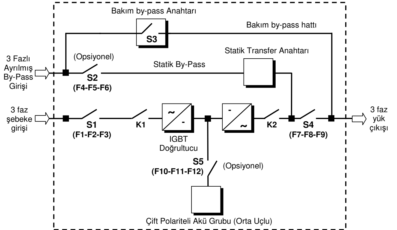
Şekil 1-2 CYCLONE 300P Serisi KGK Ayrılmış (Harici) By-Pass Blok Şeması
