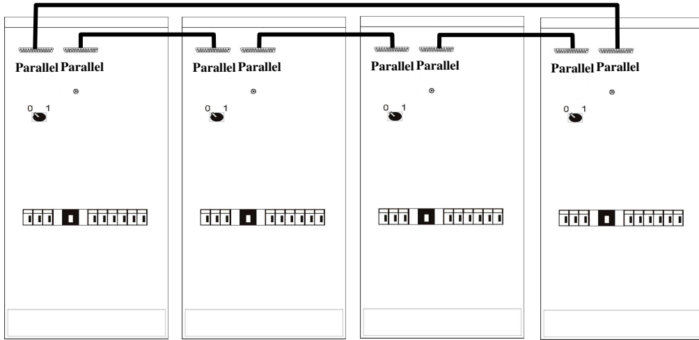
Şekil 4.2.c Dört KGK'nın Paralel ağılantısı
