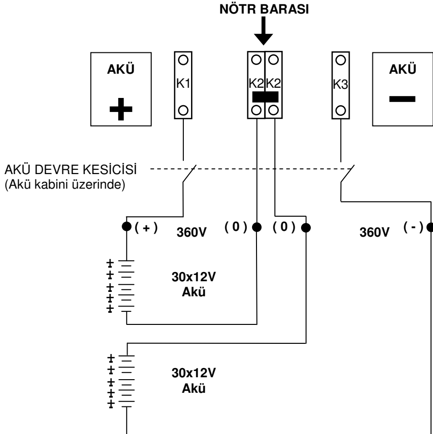
Şekil 2.3 Akü Bağlantısı (60x12V)
