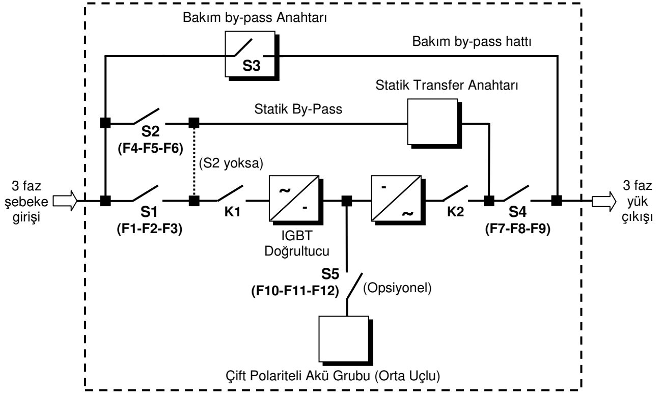
Şekil 1.1 CYCLONE 300P Serisi KGK Blok
