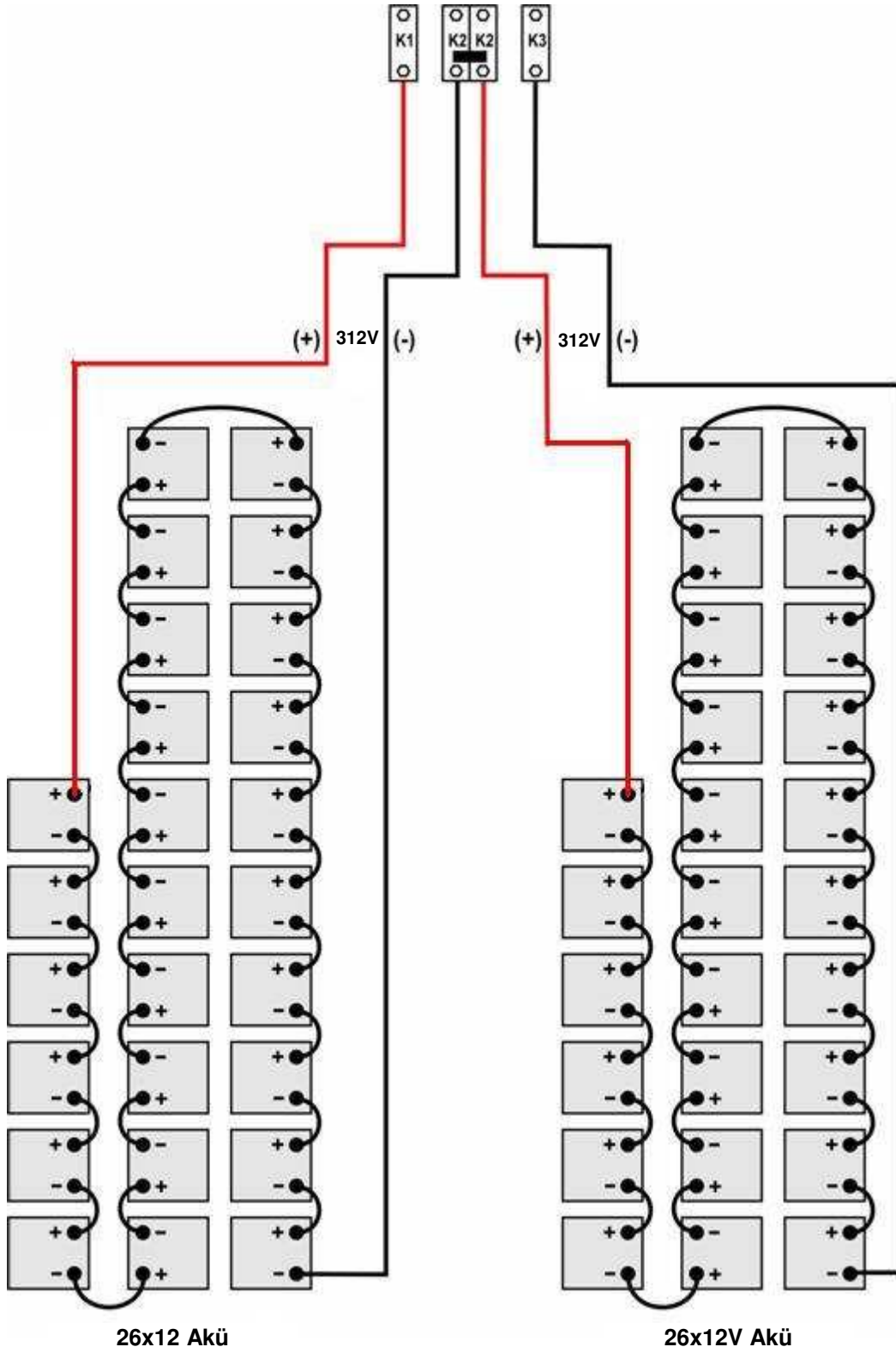
Figure 2.4 60-80 KVA Akü Yapılandırma
