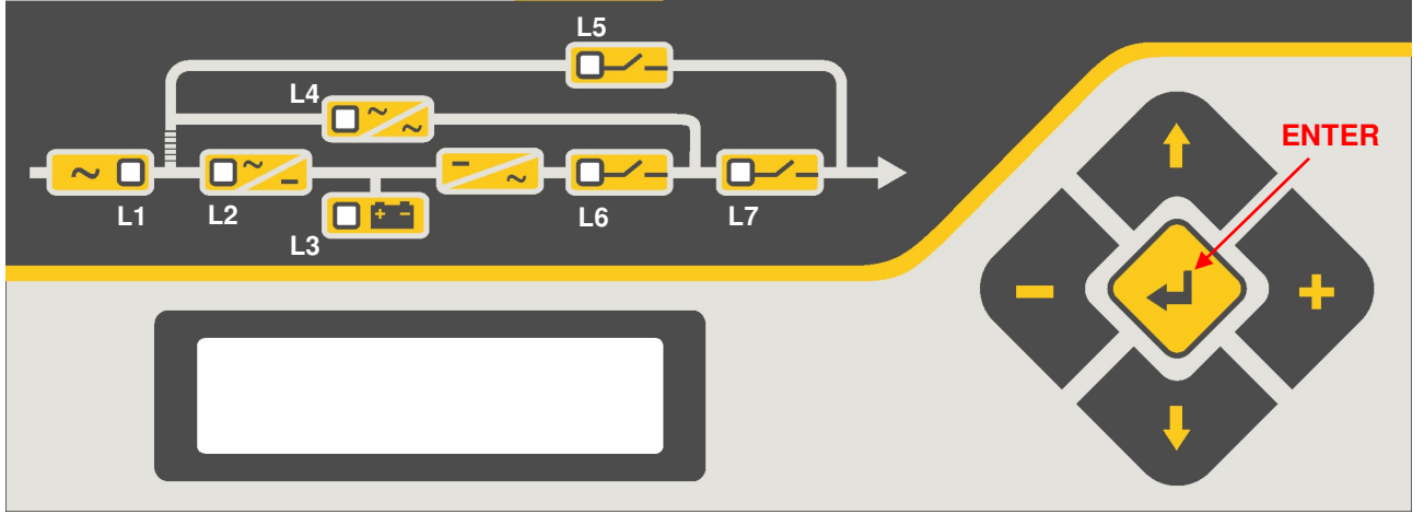
Şekil 3.1 Operatör kontrol ve gösterge paneli
