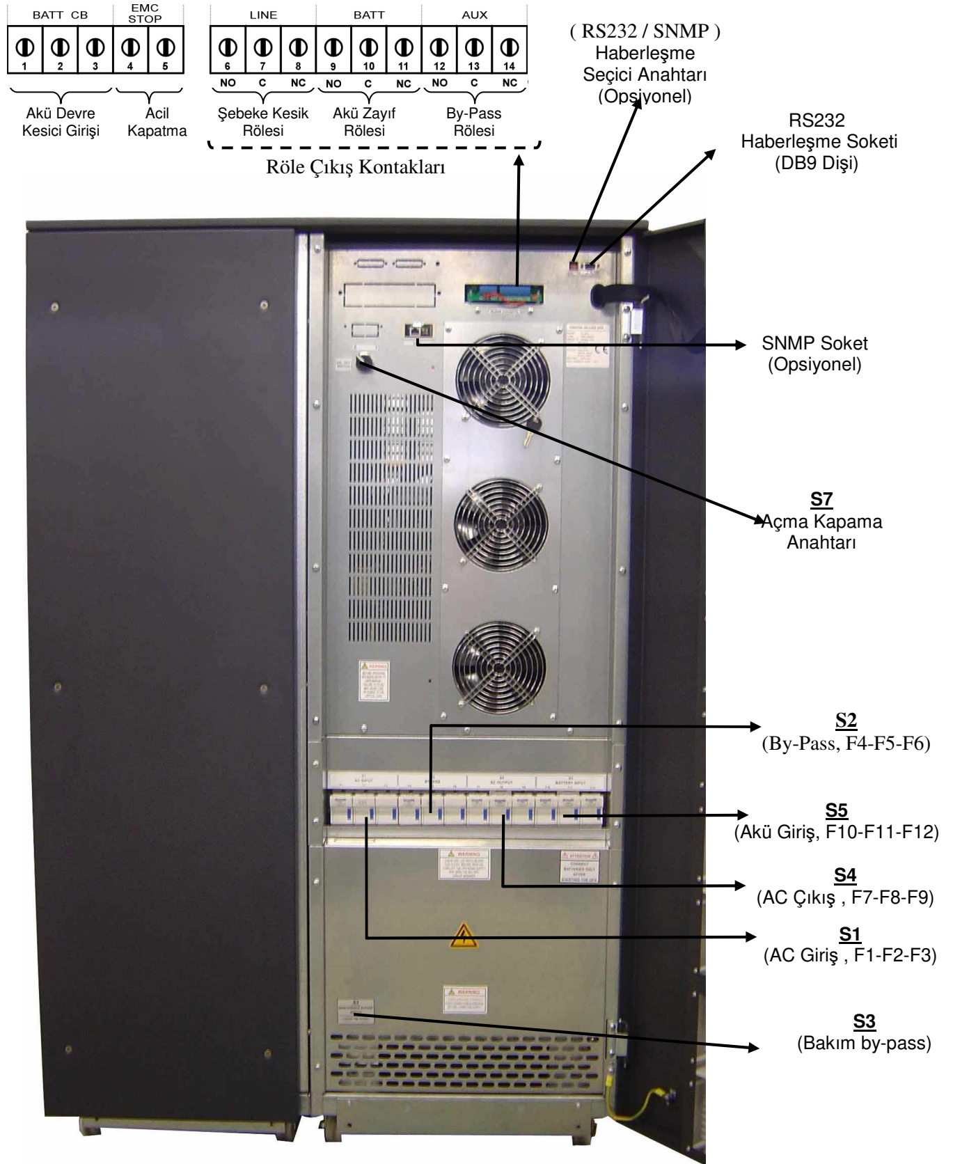
Figure 1.2 60-80 kVA Switch Yapılandırma
