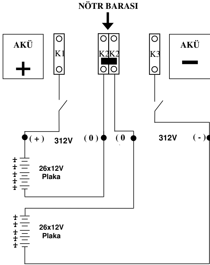
Şekil 2.3 Akü Bağlantıları (52x12V)
