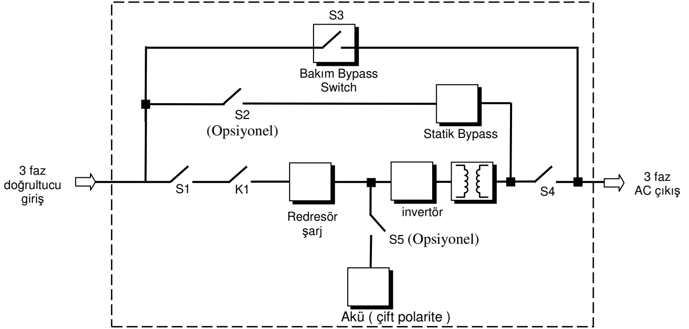
Şekil 1.1 CYCLONE 300T Serisi UPS Blok Şeması
