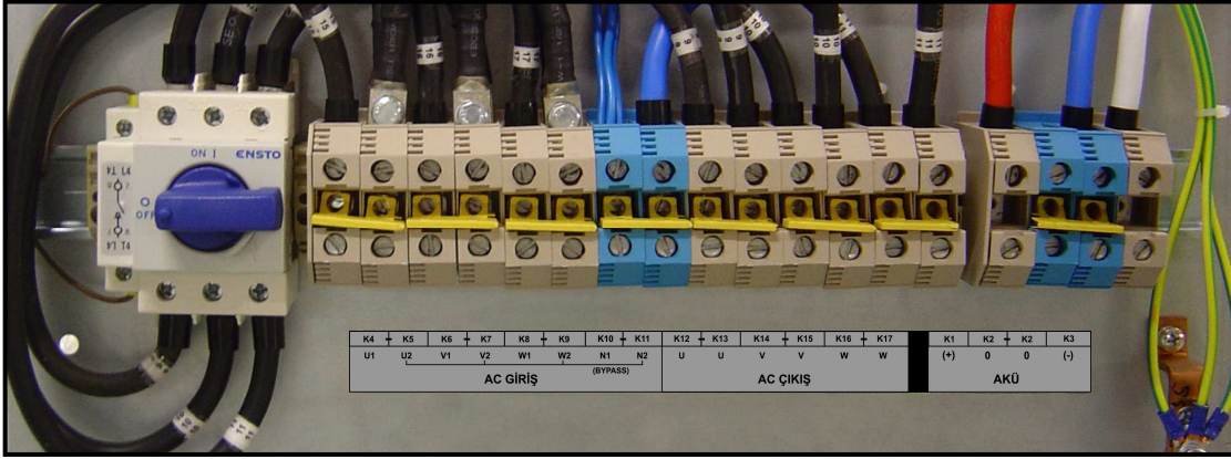
Şekil 2.2.b 60-80kVA Kablo Bağlantısı
